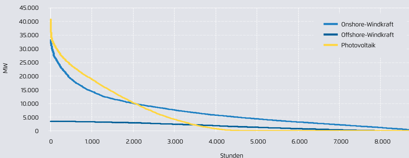
Jahresdauerlinien für dargebotsabhängige Erzeugungstechnologien (Unteres Erlösszenario), 2015
