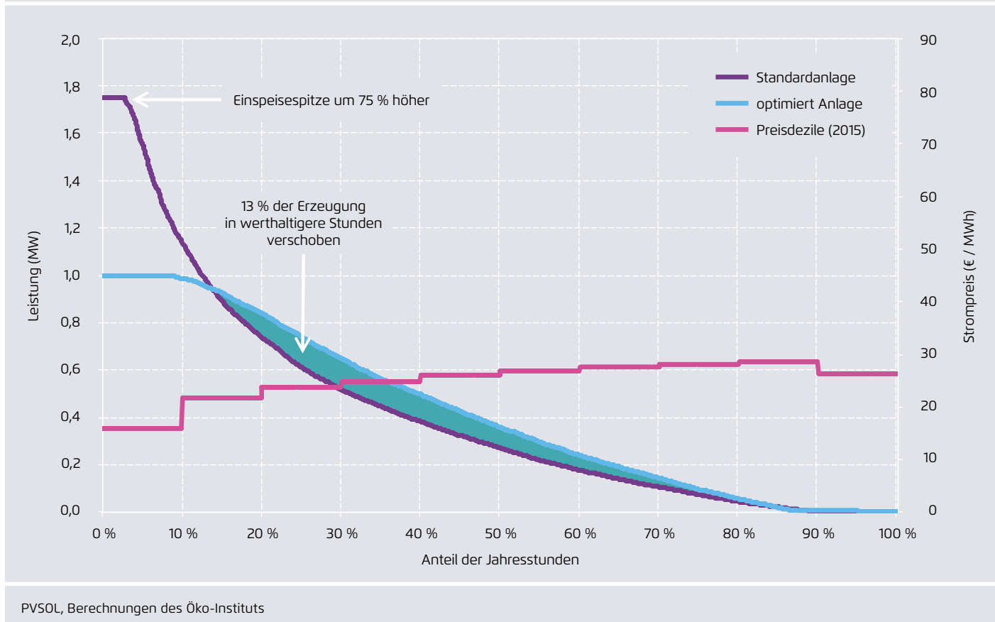
Vergleich der Jahresdauerlinien der Standardanlage und der optimierten Anlage für den Standort Stade bei gleicher Stromerzeugung beider Anlagen mit dem durchschnittlichen Strompreis
