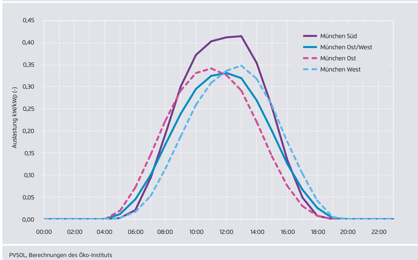
Jahresdurchschnittlicher täglicher Leistungsgang der Photovoltaikanlagen (München)
