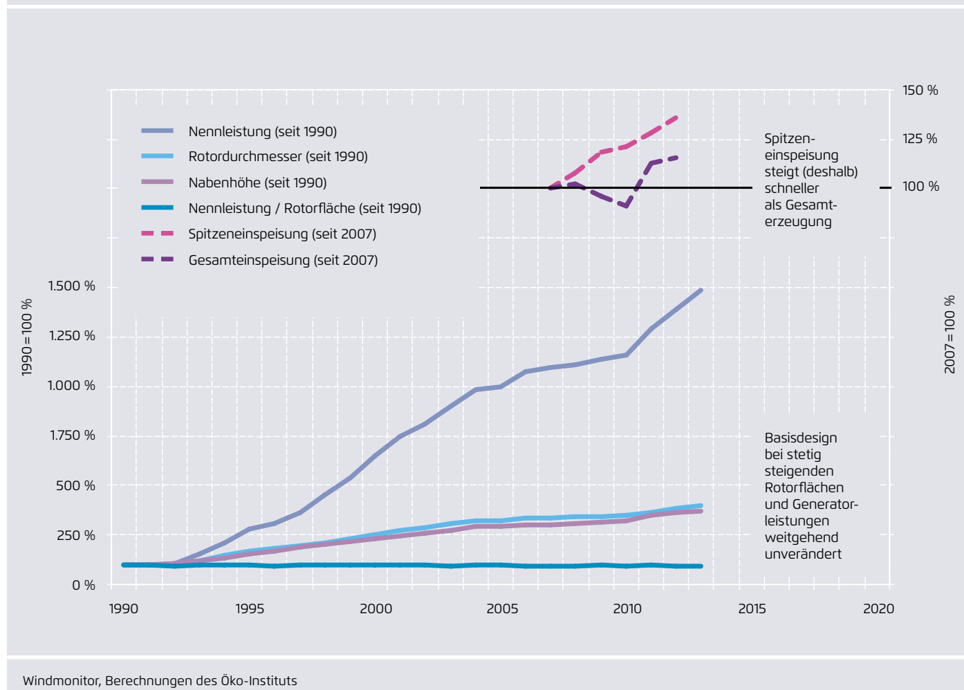
Entwicklung wichtiger Indikatoren für die Auslegung von Windkraftanlagen in Deutschland, 1990 bis 2013
