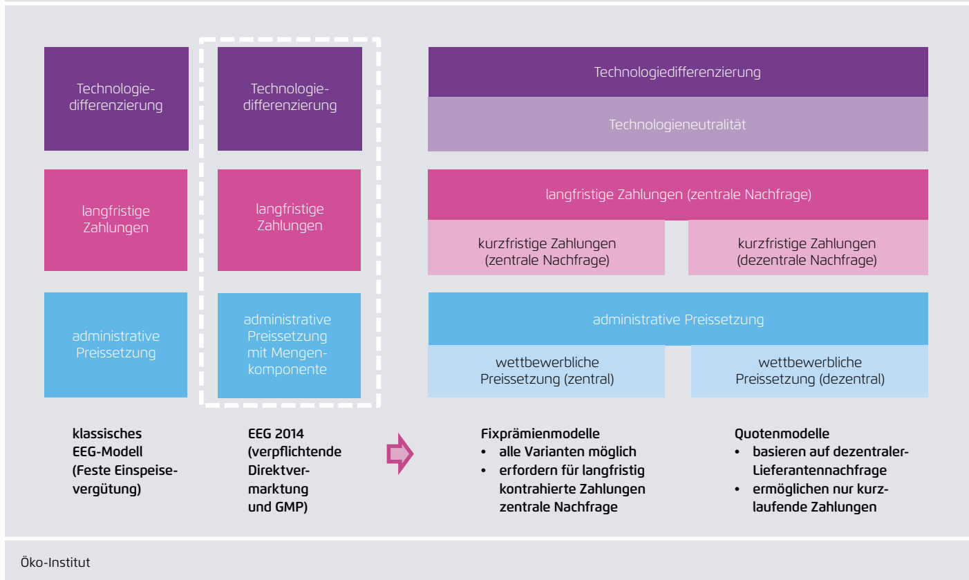
Übersicht zu den Parametrisierungsvarianten der aktuell diskutierten Reformvorschläge
