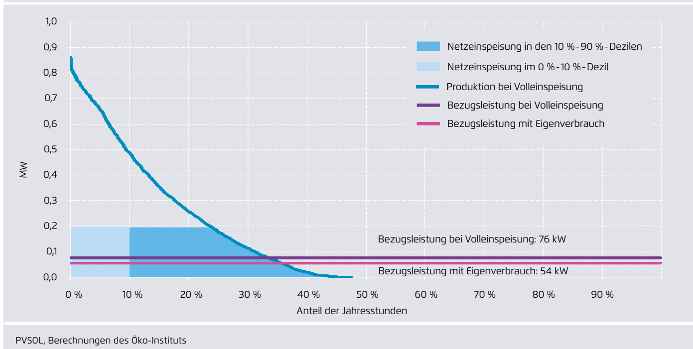
Beispielhafte Wirkung eines systemdienlich strukturierten Eigenverbrauchs auf die Jahresdauerlinie der Einspeisung und die sich daraus ergebende Bezugsleistung für die Prämienzahlung
