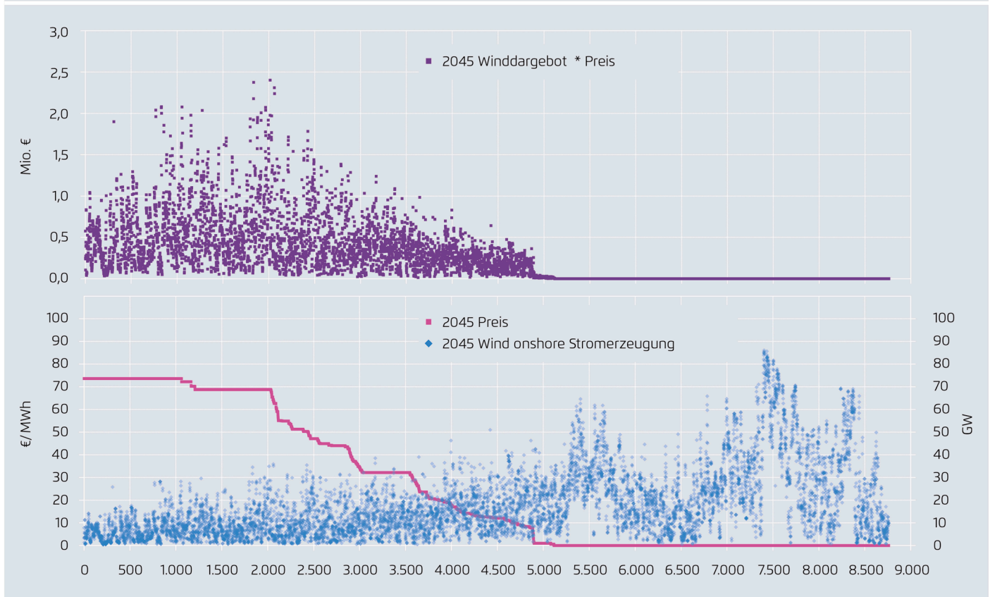
Dauerlinie der Strompreise und zugehörige Stromerzeugung sowie Erlöse für Onshore-Windenergie im Unteren Erlösszenario 2045
