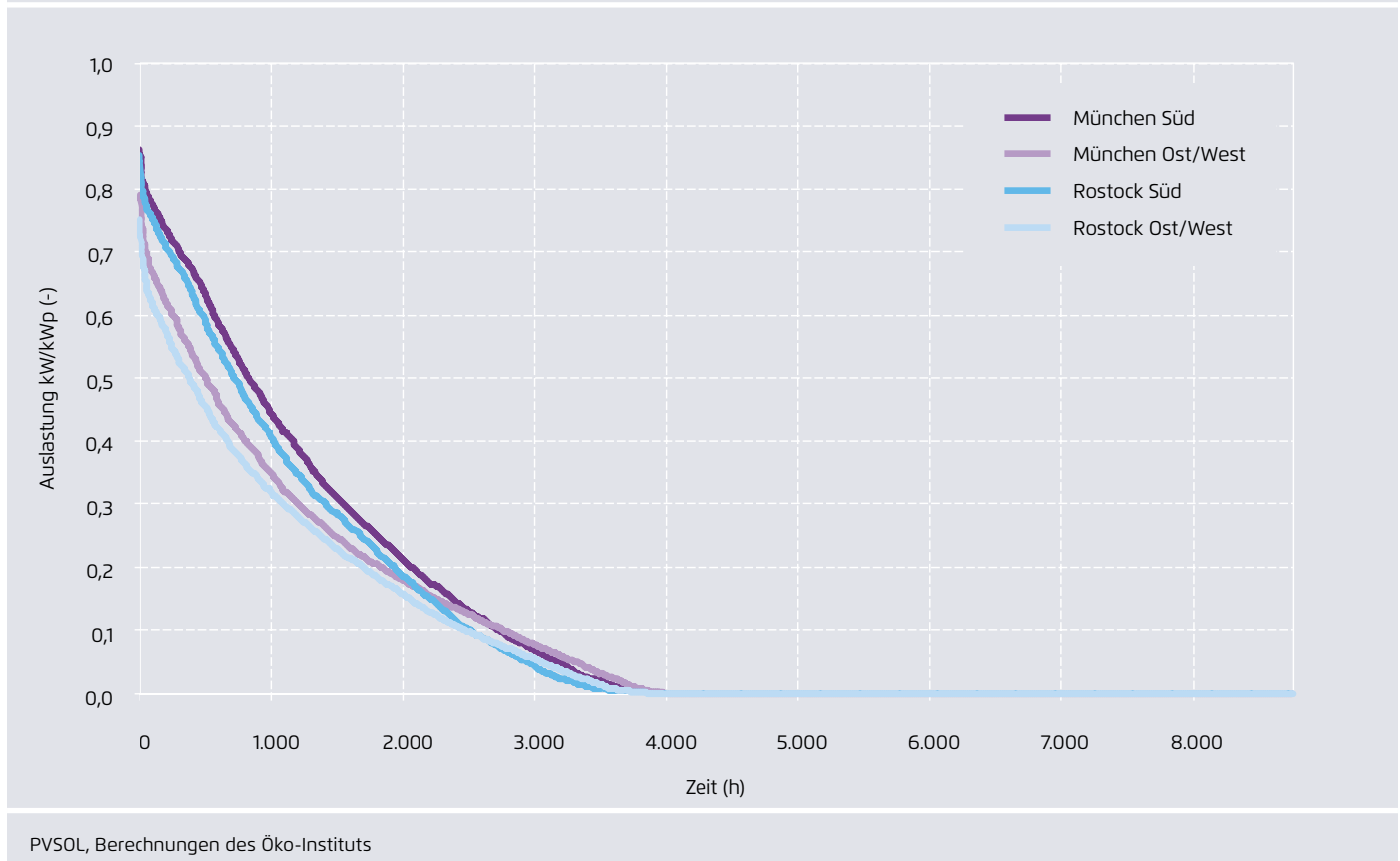
Geordnete Jahresdauerlinien der Auslastung für die betrachteten Photovoltaikanlagen
