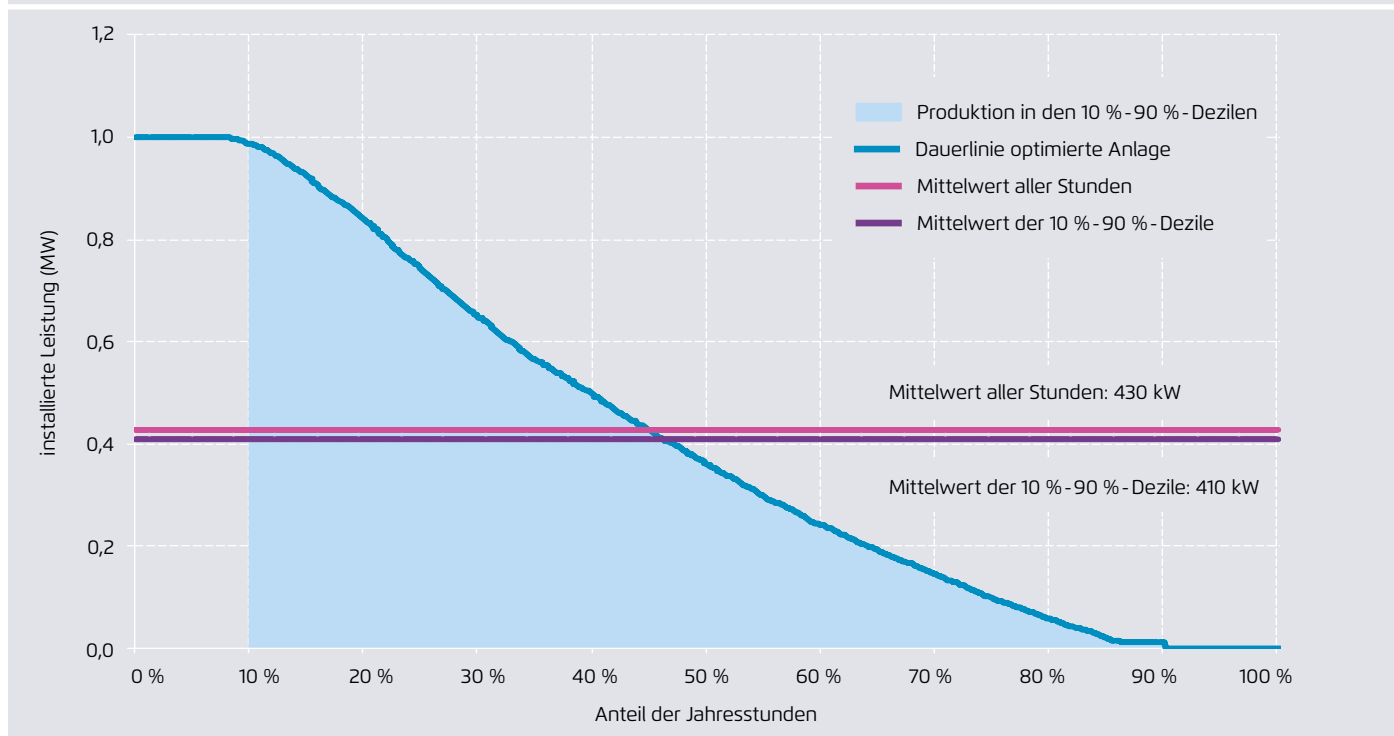
Geordnete Jahresdauerlinien der optimierten Windkraftanlage am Standort Magdeburg, 2012
