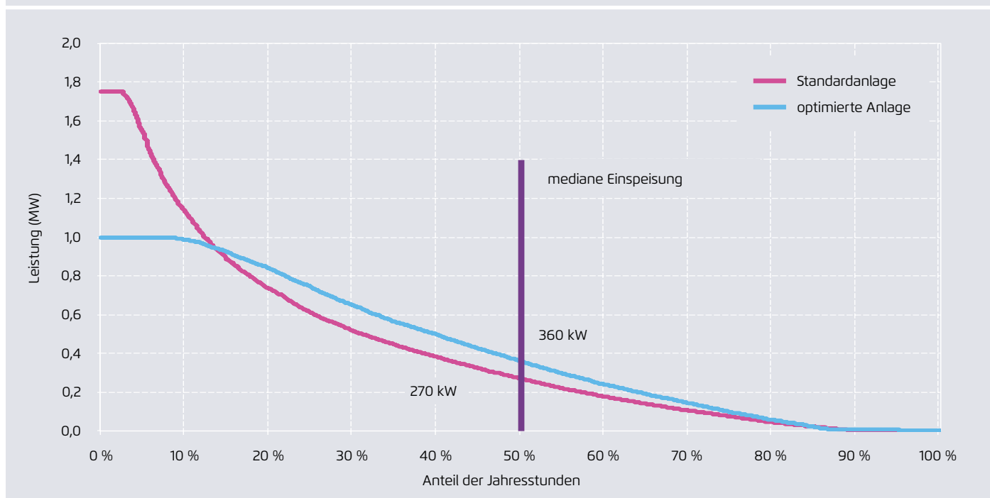
Geordnete Jahresdauerlinien der betrachteten Windkraftanlagen am Standort Stade, 2012
