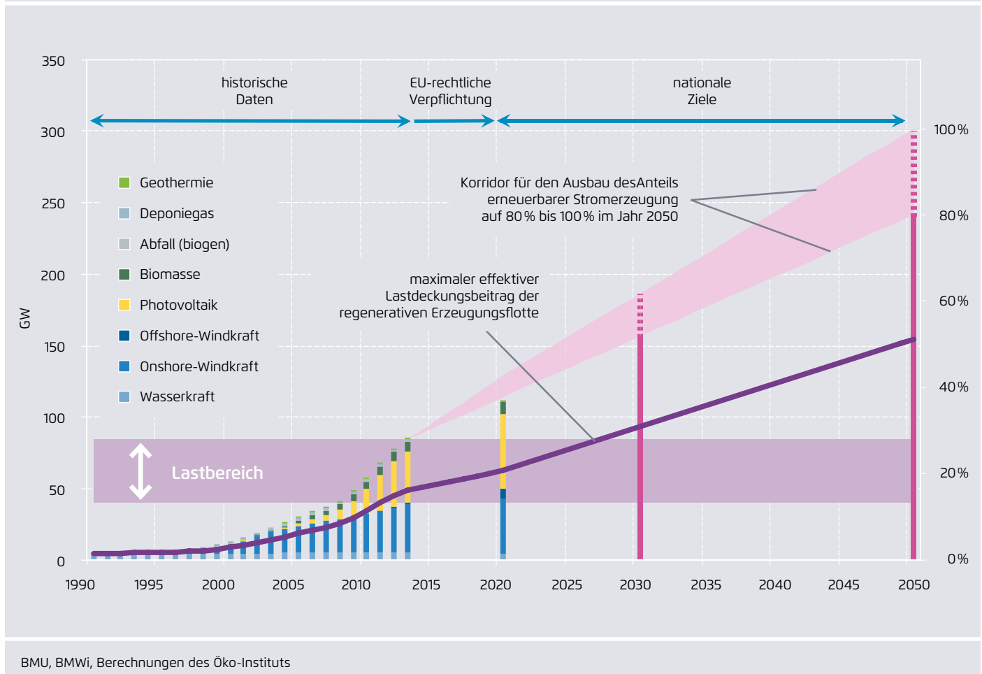
Historische und zielkonforme Entwicklung der Stromerzeugungskapazitäten auf Basis Erneuerbarer Energien, 1990 bis 2050
