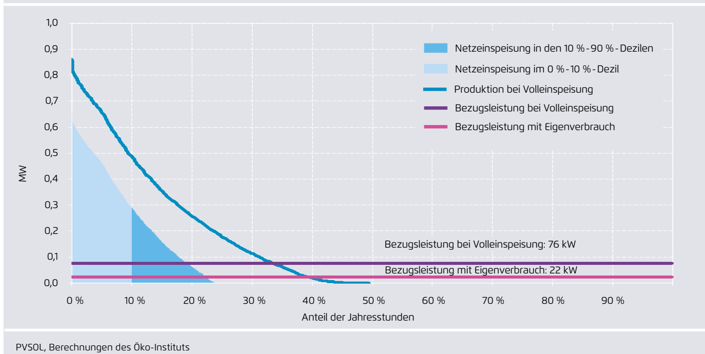
Beispielhafte Wirkung einer nicht systemdienlichen Strukturierung des Eigenverbrauchs auf die Jahresdauerlinie der Einspeisung und sich daraus ergebende Bezugsleistung für die Prämienzahlung
