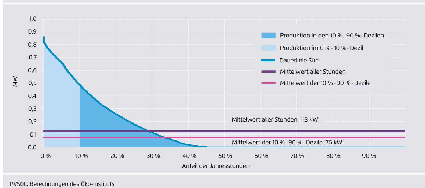
Bestimmung der Bezugskapazität für Photovoltaikanlagen
