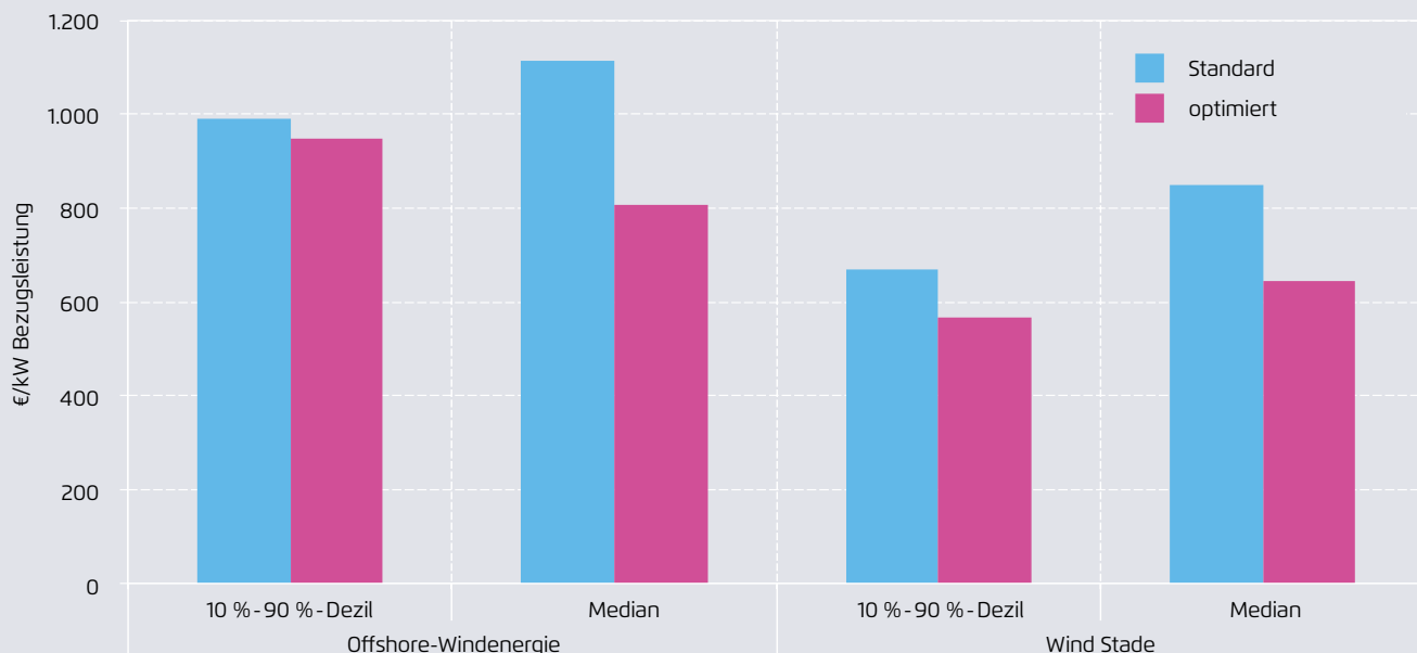
Kapazitätsprämien für Windkraftanlagen: Vergleich von Median- und Dezilmethode zur Berechnung der Bezugsleistung
