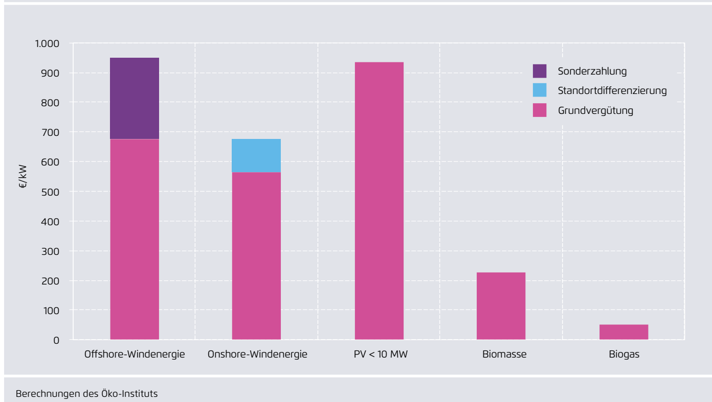
Vergleich der Höhe der Kapazitätsprämie im Jahr 2015 (für die jeweiligen Bezugsleistungen)
