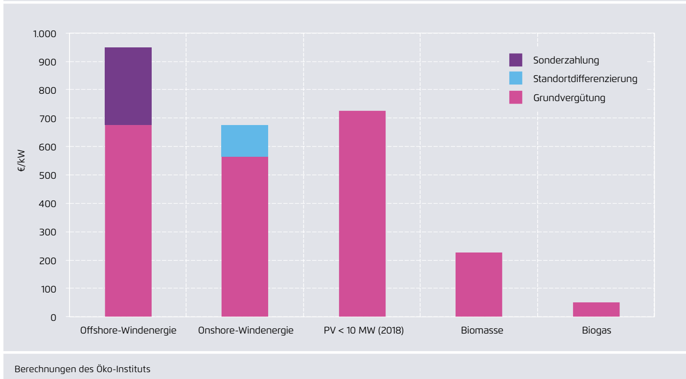
Vergleich der Höhe der Kapazitätsprämie in der Perspektive (10-Prozent-/90-Prozent-Dezile)
