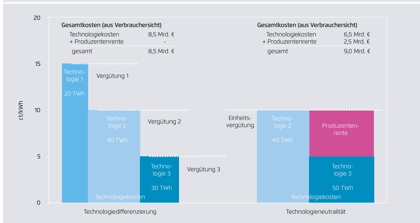
Spannungsfeld von Technologiekosten und inframarginalen Verteilungseffekten bei technologie-differenzierten und technologie-neutralen Ansätzen
