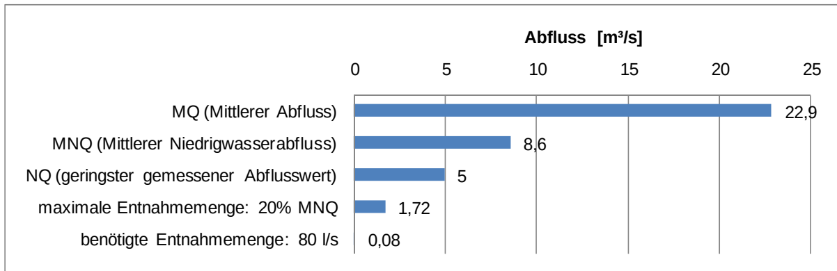
Abbildung 5: Abflussverhältnisse der Loisach (MQ, MNQ und NQ) im Vergleich zur Vorgabe der maximalen und der tatsächlich benötigten Entnahmemenge
