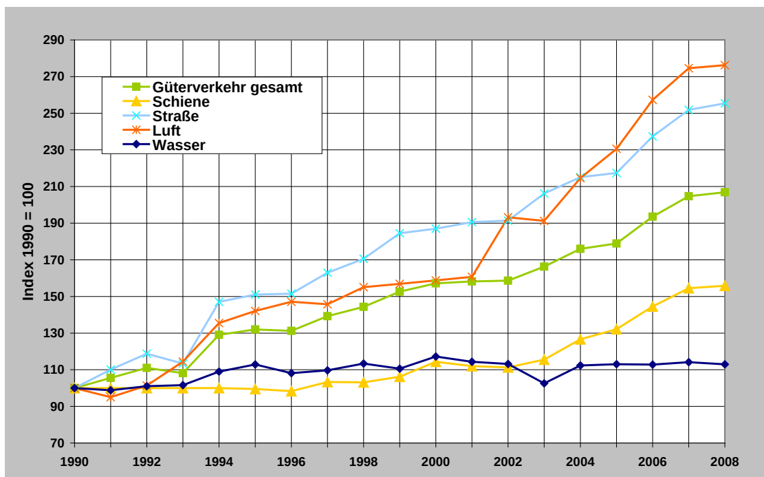
Abbildung 6-7 Entwicklung Verkehrsleistung Güterverkehr 36
