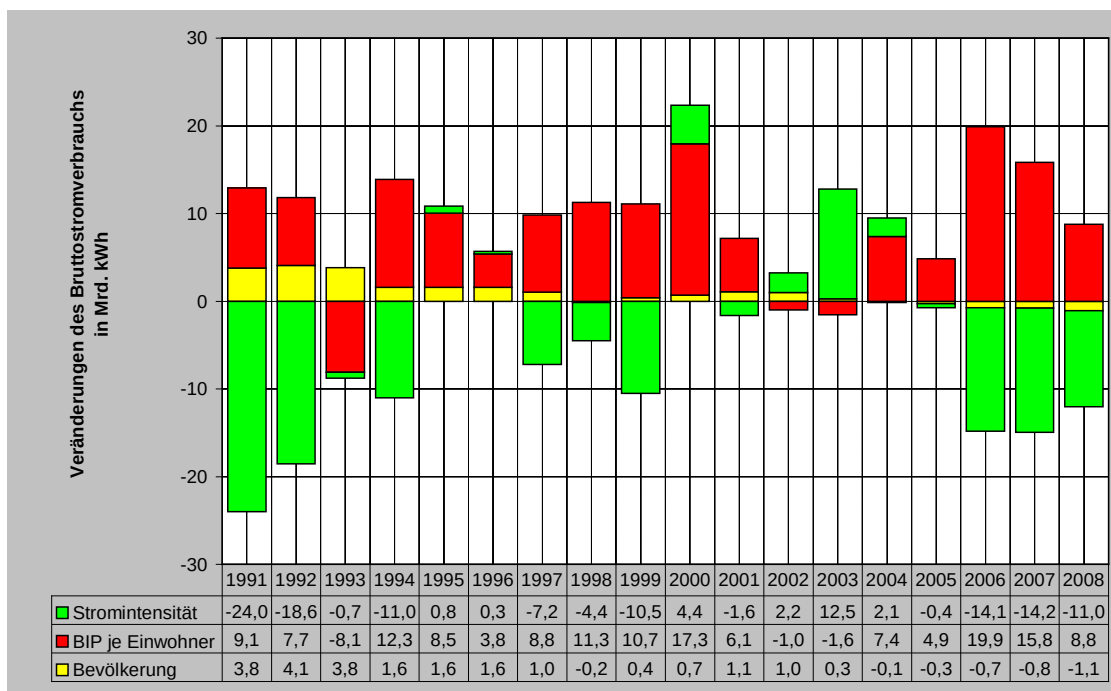
Abbildung 7-8 Beiträge verschiedener Einflussfaktoren zu den jährlichen Veränderungen des Bruttostromverbrauchs in Deutschland von 1990 bis 2008
