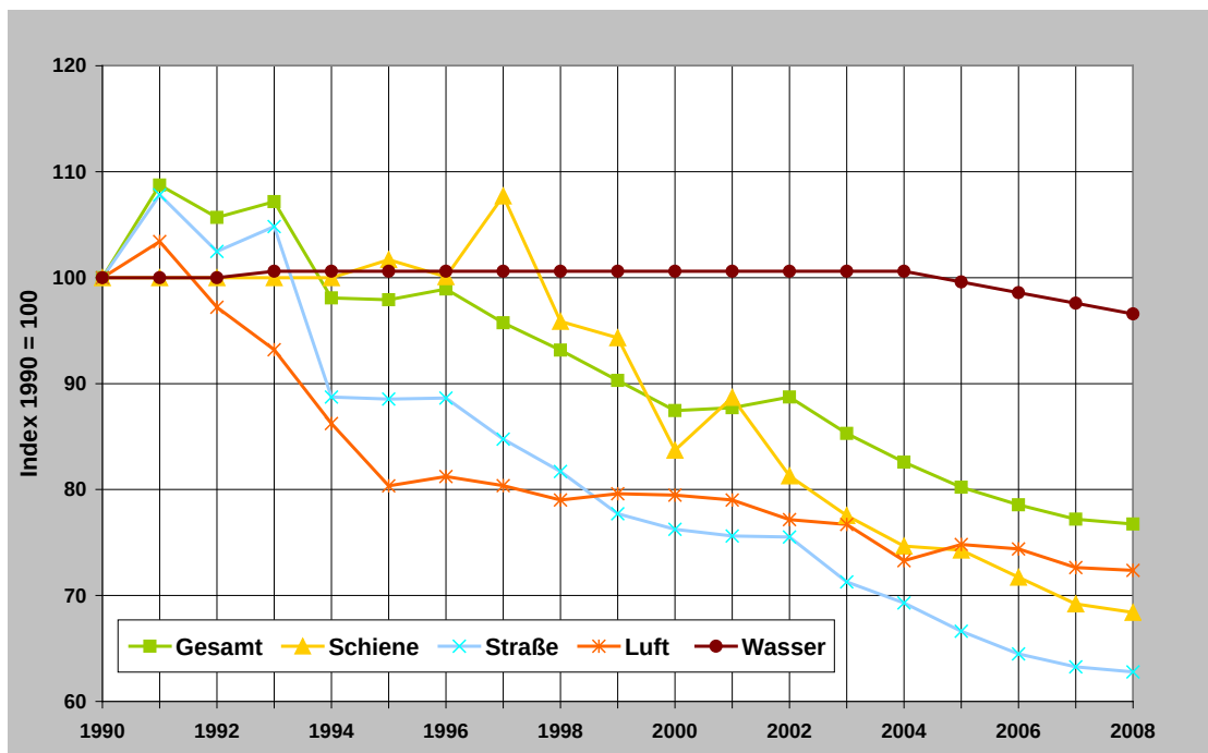
Abbildung 6-2 Entwicklung Endenergieverbrauch Güterverkehr 34 (Endenergieverbrauch bezogen auf die Verkehrsleistung)
