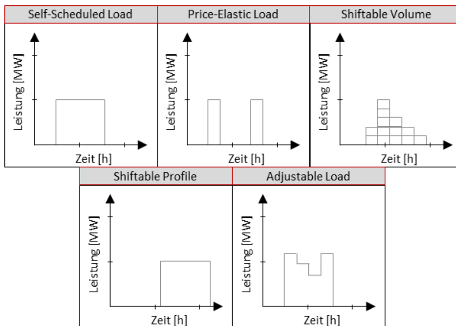
Abbildung 8: Nachfrageseitige Gebotsformen
