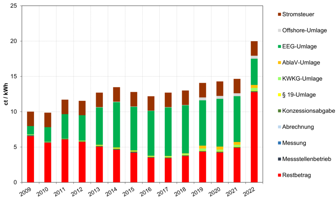
Abbildung 12: Entwicklung Industriestrompreise
