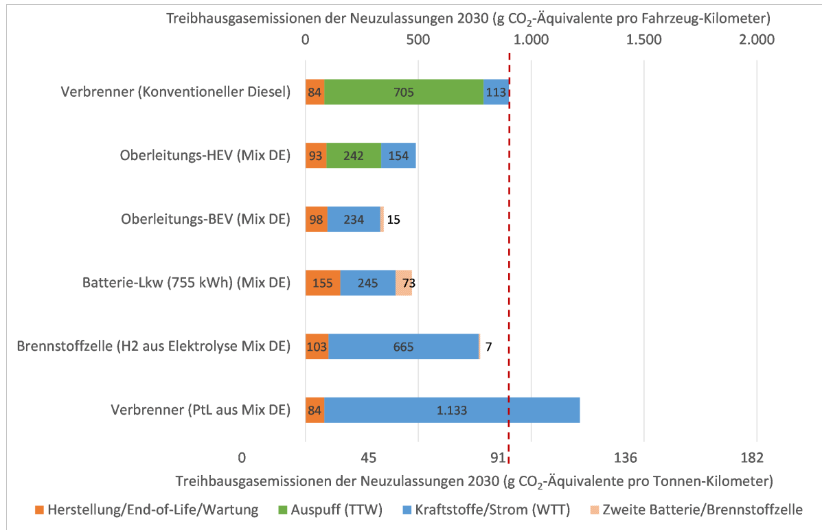
Abbildung 2: Treibhausgasemissionen 2030 zugelassener Sattelzugmaschinen (40 t zGG) mit verschiedenen Antriebskonzepten für typische Nutzungsparameter in Deutschland (800.000 km Laufleistung über 7 Jahre Betriebsdauer, 11 t durchschnittliche Zuladung, Deutscher Strommix). Quelle: Helms 2022
