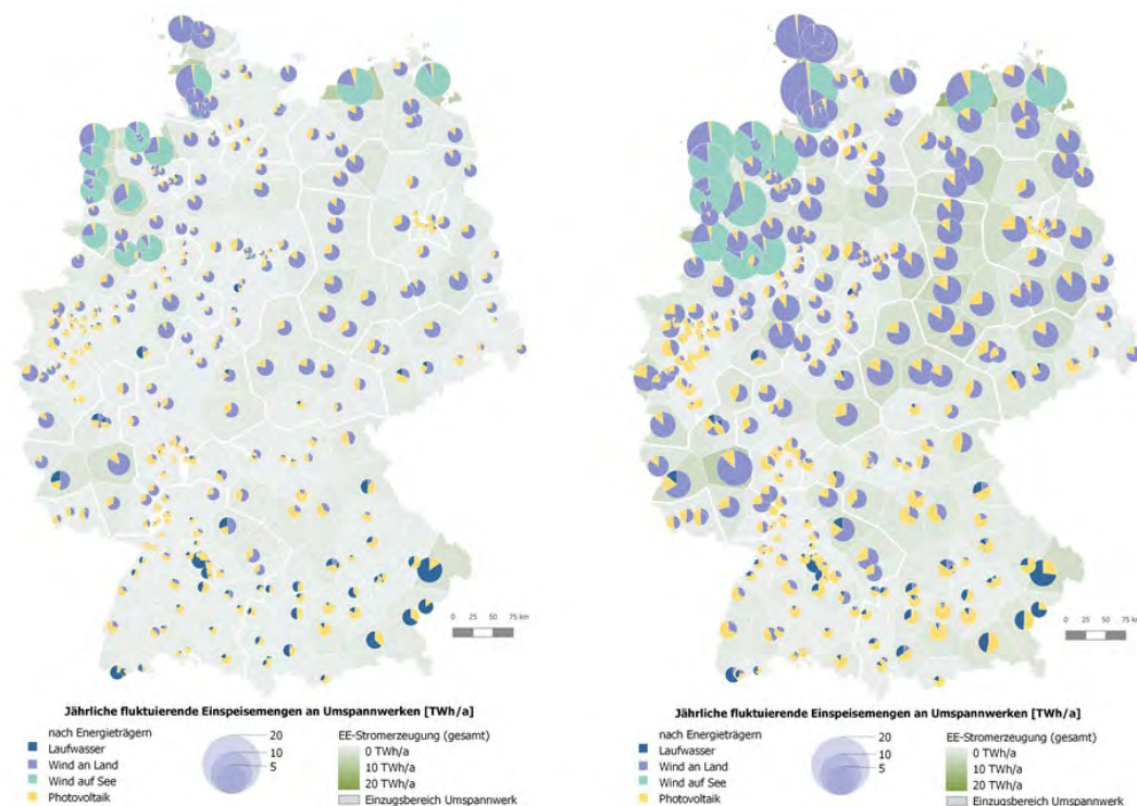
Abbildung 7.7-18: Regionalisiertes EE-Stromangebot je Übertragungsnetzknotten in den Szenarien „Enera Worst Case 2030“ (links) und „Enera Best Case 2050“ (rechts)
