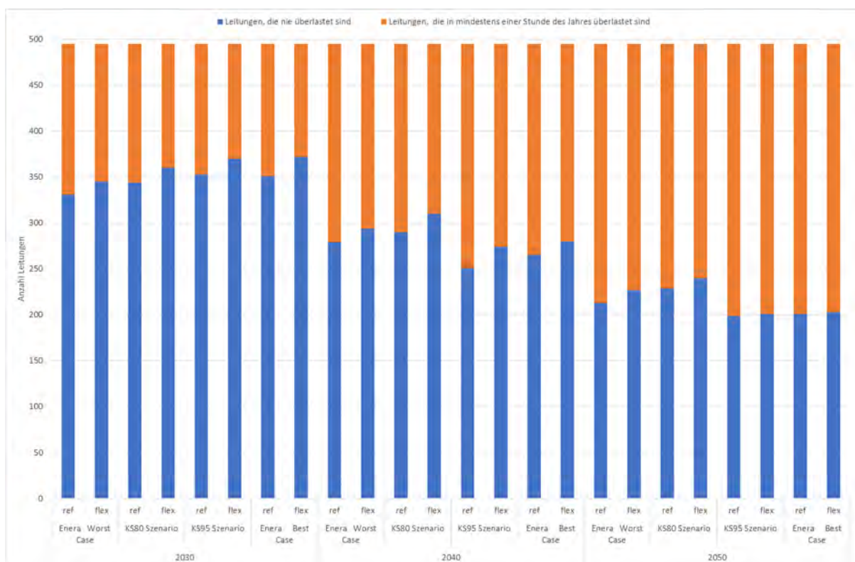
Abbildung 7.7-21: Anzahl der überlasteten Leitungen in den enera Szenarien vor („ref“) und nach („flex“) dem übertragungsnetzdienlichen Einsatz von dezentraler Flexibilität
