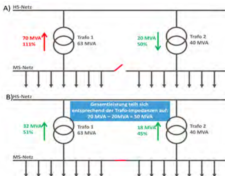
Abbildung 6.1-2: Beispiel für die Kopplung von Mittelspannungsnetzen
