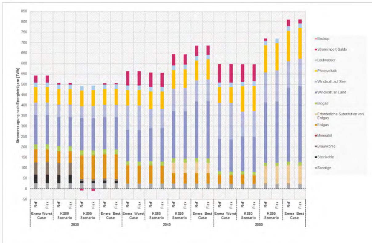
Abbildung 7.7-3: Strommix in Deutschland vor („ref“) und nach („flex“) dem strommarktdienlichen Einsatz der dezentralen Flexibilitätsoptionen
