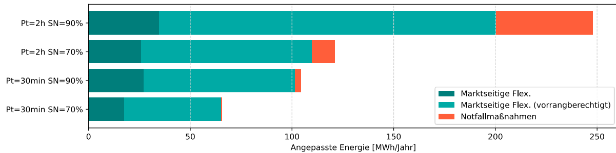
Abbildung 6.2-4: Umgesetzte Wirkleistungs-Anpassungsmaßnahmen im gesamten Jahr in Abhängigkeit des Prognosehorizonts und berücksichtigten Sicherheitsniveaus
