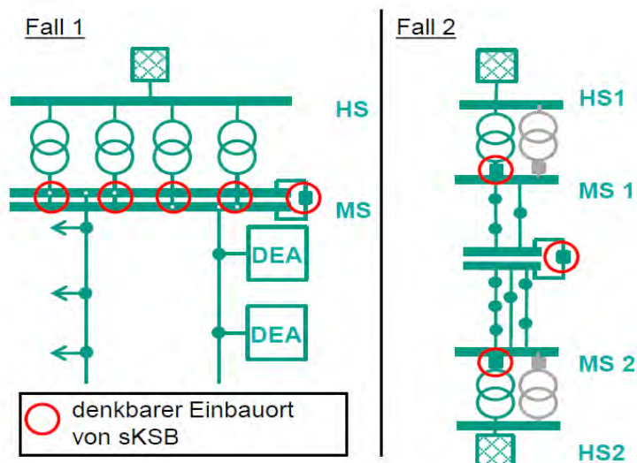
Abbildung 6.1-1: Nutzungsfälle von sKSB zur Netzkopplung
