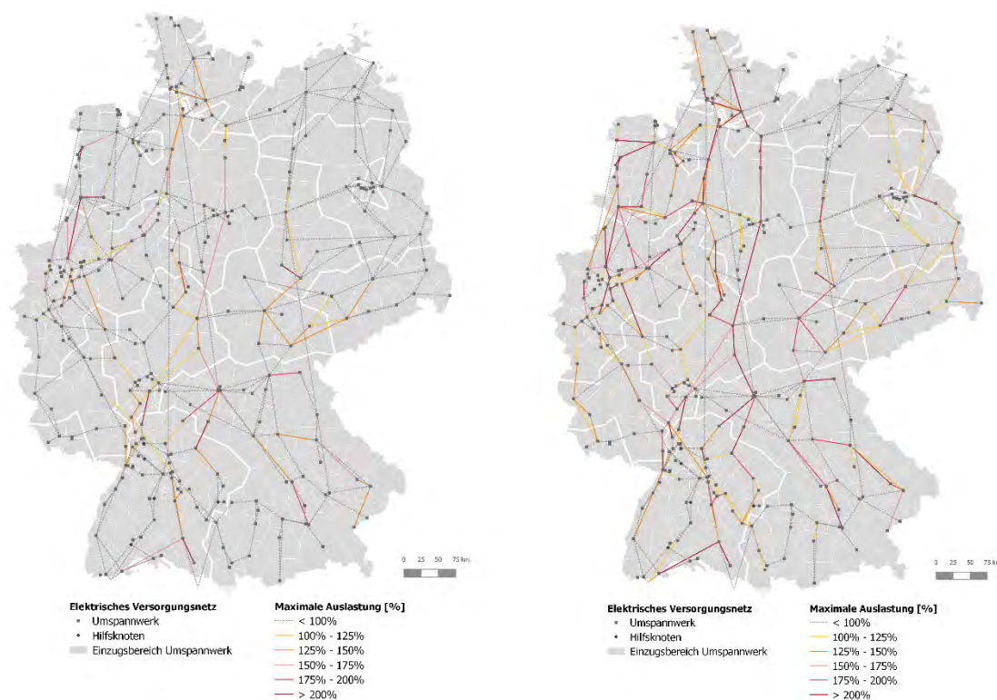
Abbildung 7.7-25: Maximale Überlastung auf den einzelnen Leitungen in den Referenzszenarien „Enera Worst Case 2030“ (links) und „Enera Best Case 2050“ (rechts)
