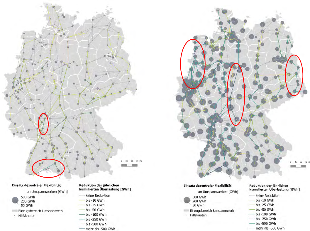
Abbildung 7.7-26: Reduktion der kumulierten Überlastung auf den einzelnen Leitungen durch den übertragungsnetzdienlichen Einsatz dezentraler Flexibilität in den Szenarien „Enera Worst Case 2030“ (links) und „Enera Best Case 2050“ (rechts)
