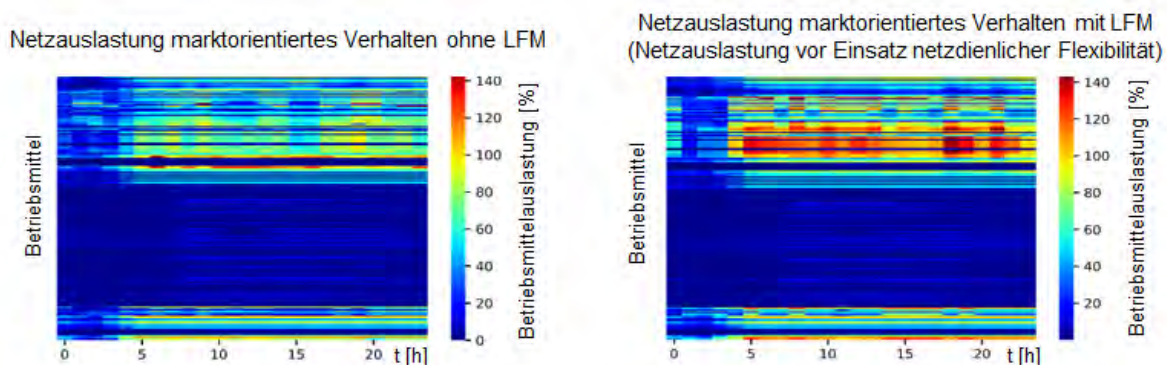
Abbildung 6.2-7: Netzauslastung nach Lernprozess bei Vermarktungsmöglichkeit am Spotmarkt (links) und Netzauslastung nach Lernprozess bei Vermarktungsmöglichkeit am Spot- und Flexmarkt (rechts)
