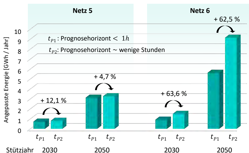
Abbildung 6.3-11: Notwendige Wirkleistungs-Anpassungsmaßnahmen in Abhängigkeit des Prognosehorizonts, Durchschnitt über beide betrachtete Szenarien (Sicherheitsniveau: 90 %, Zeitraum: 1 Jahr)
