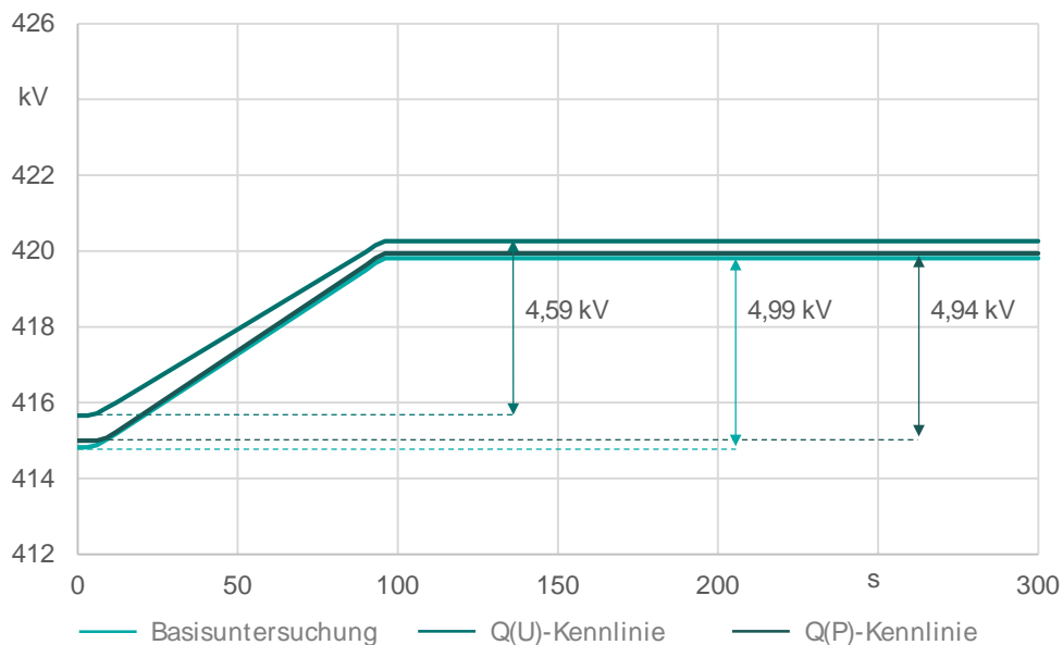
Abbildung 6.3-6: Spannungsverlauf am Fehlerort für Untersuchungsszenario 4
