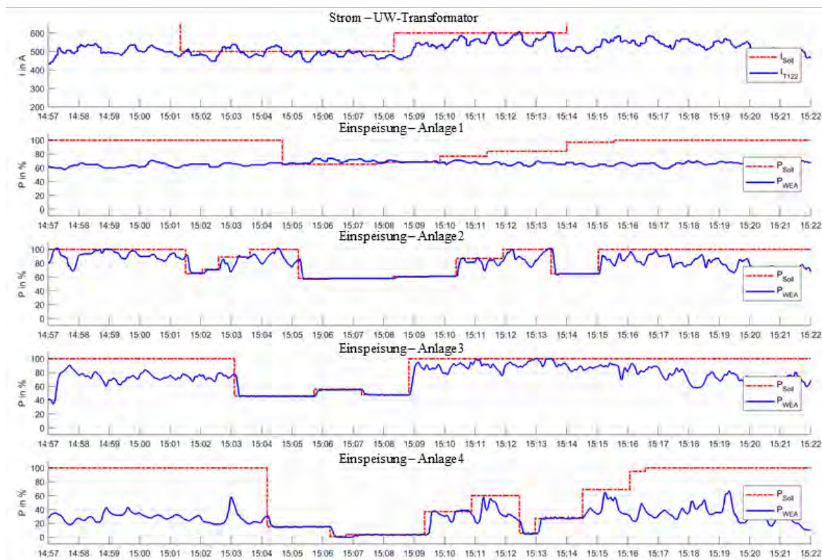
Abbildung 6.1-5: Feldtest mit dem Netzregler von Phoenix Contact im UW Wiesmoor; Transformatorstrom und Einspeiseleistungen der Erzeugungsanlagen mit dargestelltem Sollwert
