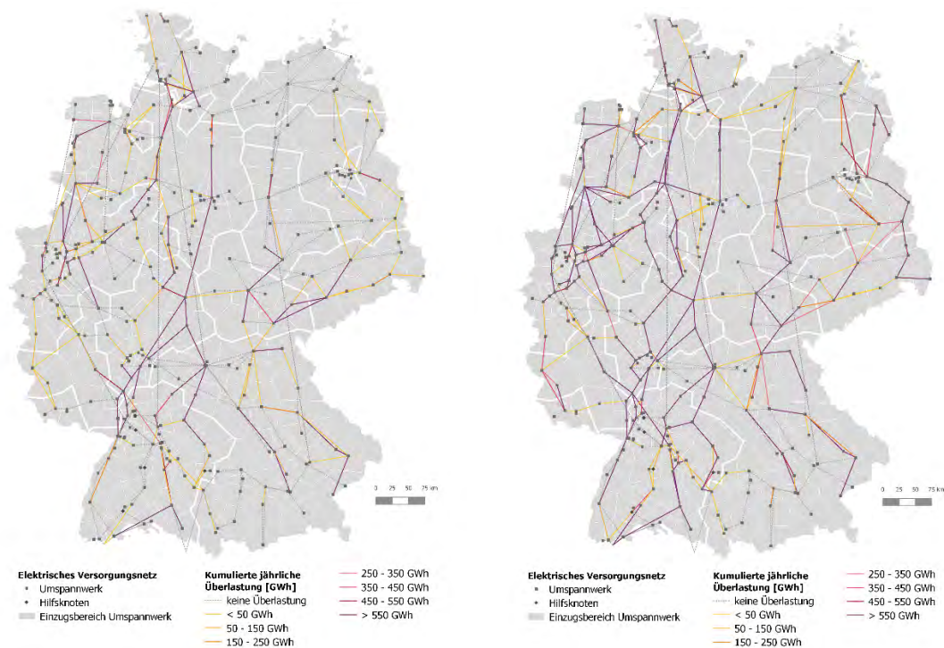
Abbildung 7.7-23: Räumliche Auflösung der kumulierten Netzüberlastung auf die einzelnen Leitungen in den Referenzszenarien „Enera Worst Case 2030“ (links) und „Enera Best Case 2050“ (rechts)
