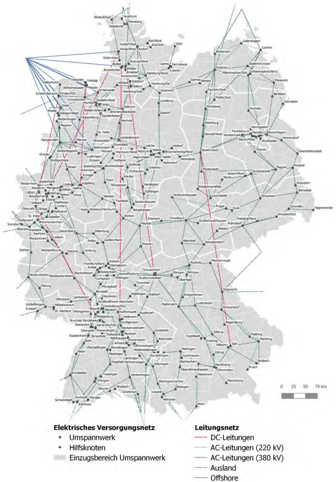
Abbildung 3.3-1: Netztopologie für das deutsche Übertragungsnetz
