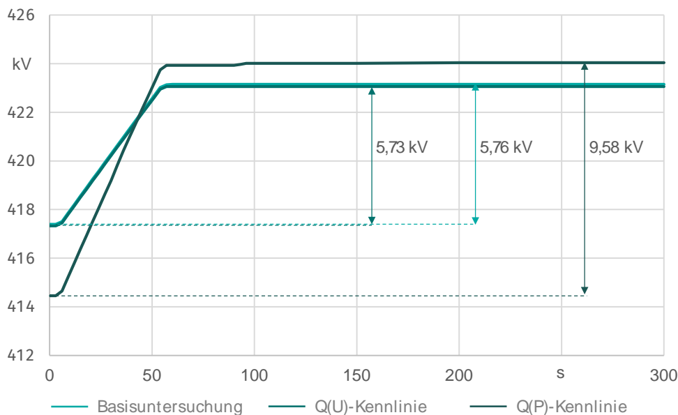
Abbildung 6.3-4: Spannungsverlauf am Fehlerort für Untersuchungsszenario 2
