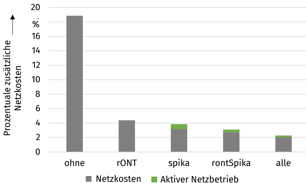
Abbildung 5.2-2: Ergebnis für die volkswirtschaftliche Bewertung des Netzentwicklungsclusters 1.4.
