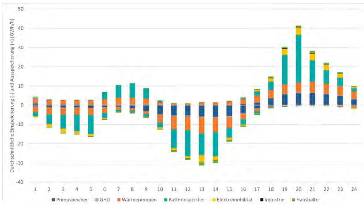
Abbildung 7.7-33: Untertägiges Be- und Entladeprofil im Best Case 2050 in GWh/h
