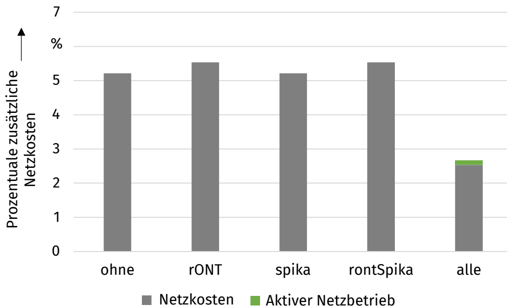
Abbildung 5.2-4: Ergebnis für die volkswirtschaftliche Bewertung des Netzentwicklungsclusters 5.1.
