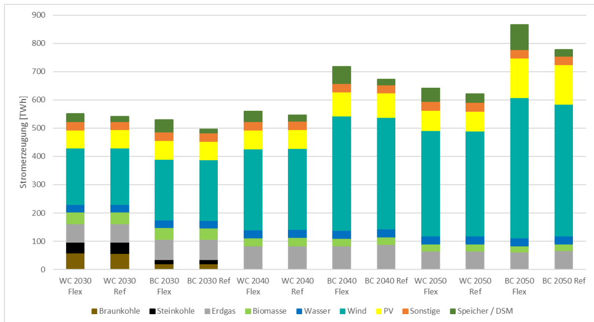
Abbildung 7.7-29: Stromerzeugungsmix in Deutschland in TWh
