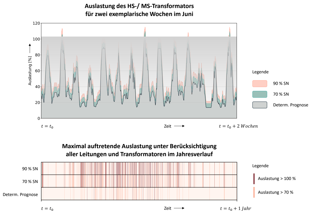
Abbildung 6.2-3: Auslastung der Netzbetriebsmittel vor Optimierung (Prognosehorizont: 30 min)
