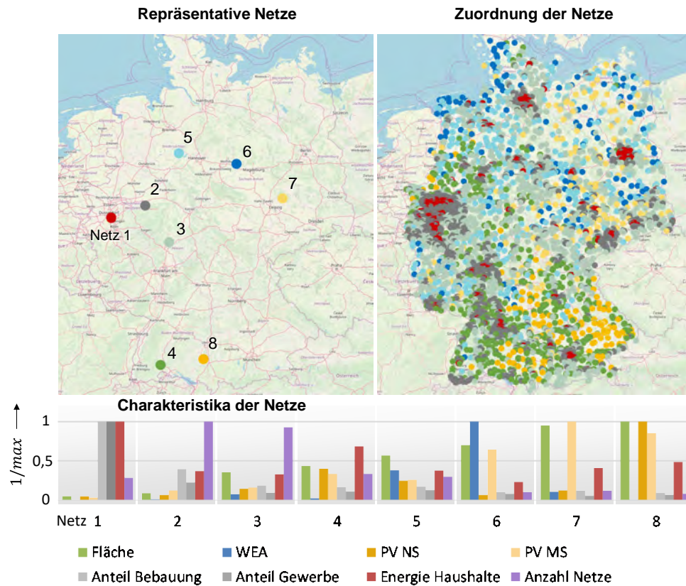
Abbildung 6.3-7: Oben links: Repräsentative Netze der Cluster, oben rechts: Zuordnung der Netze zu den Clustern, unten: Charakteristika der repräsentativen Netze
