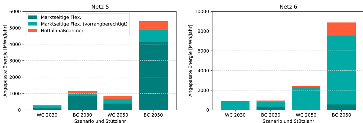
Abbildung 6.3-10: Umfang angepasster Energie nach Typ für die Netze 5 und 6 (Sicherheitsniveau: 90 %, Zeitraum: 1 Jahr)
