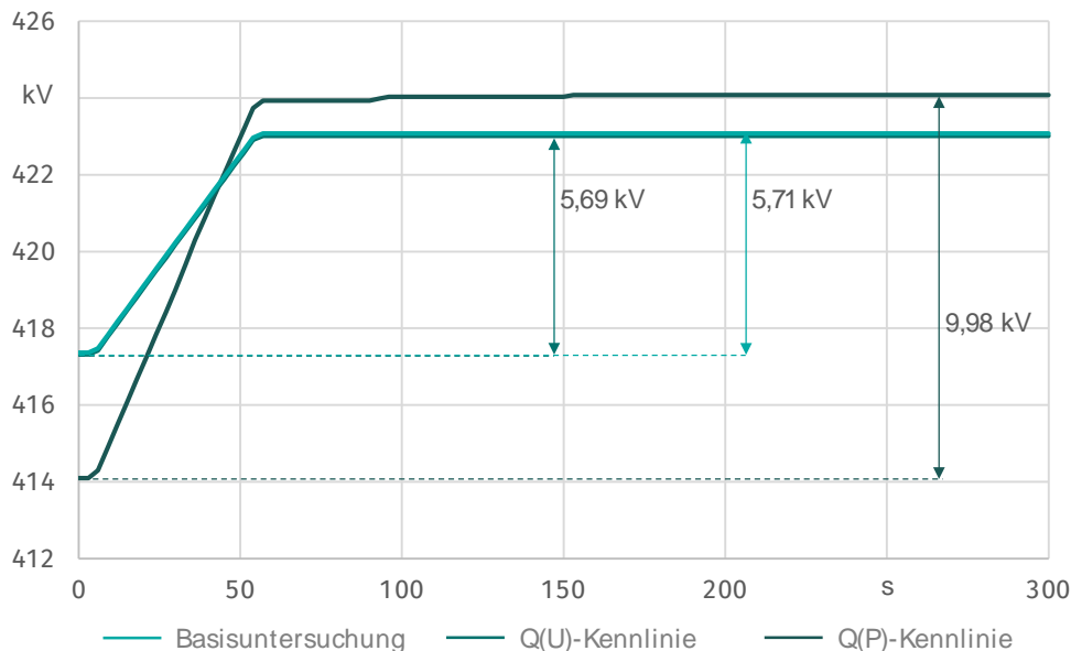
Abbildung 6.3-3: Spannungsverlauf am Fehlerort für Untersuchungsszenario 1
