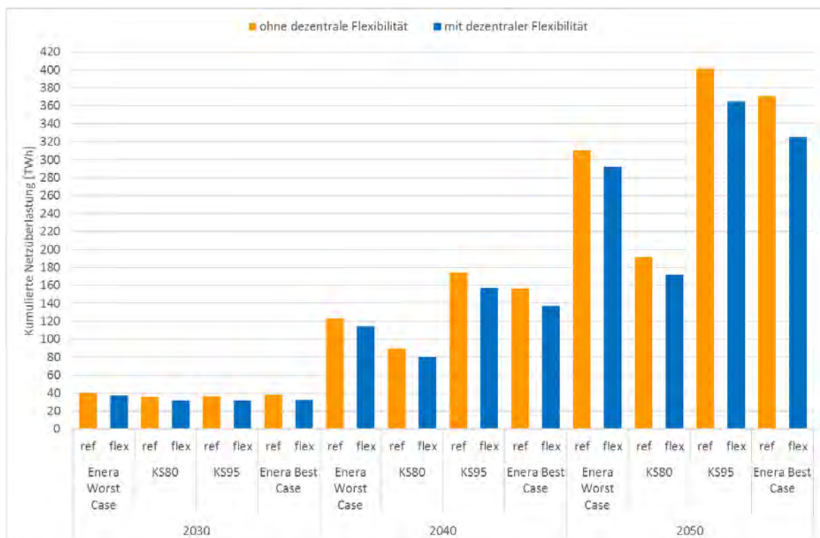
Abbildung 7.7-20: Kumulierte Netzüberlastung in den enera Szenarien vor („ref“) und nach („flex“) dem übertragungsnetzdienlichen Einsatz von dezentraler Flexibilität
