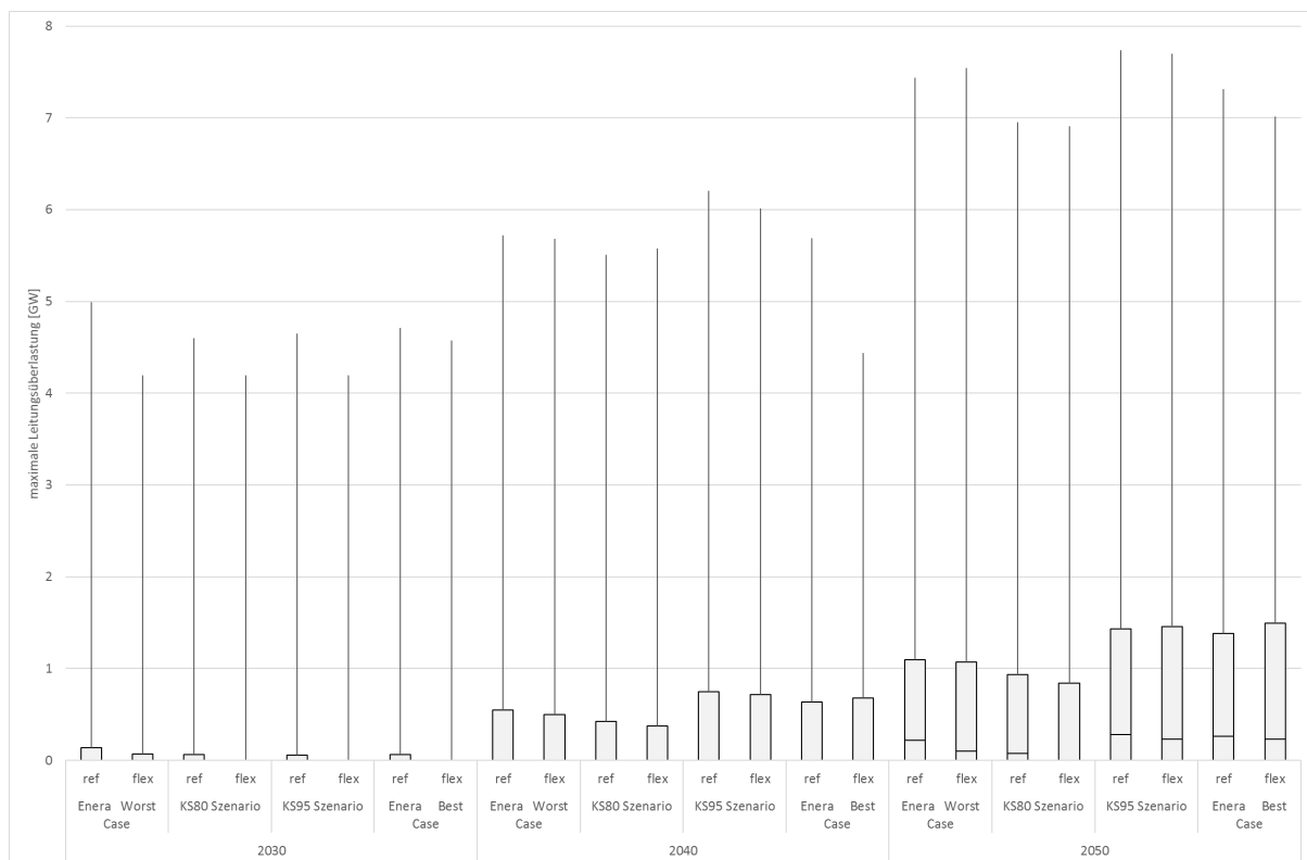
Abbildung 7.7-22: Box-Plot der maximalen Leitungsüberlastung für alle AC-Leitungen in den enera Szenarien vor („ref“) und nach („flex“) dem übertragungsnetzdienlichen Einsatz von dezentraler Flexibilität
