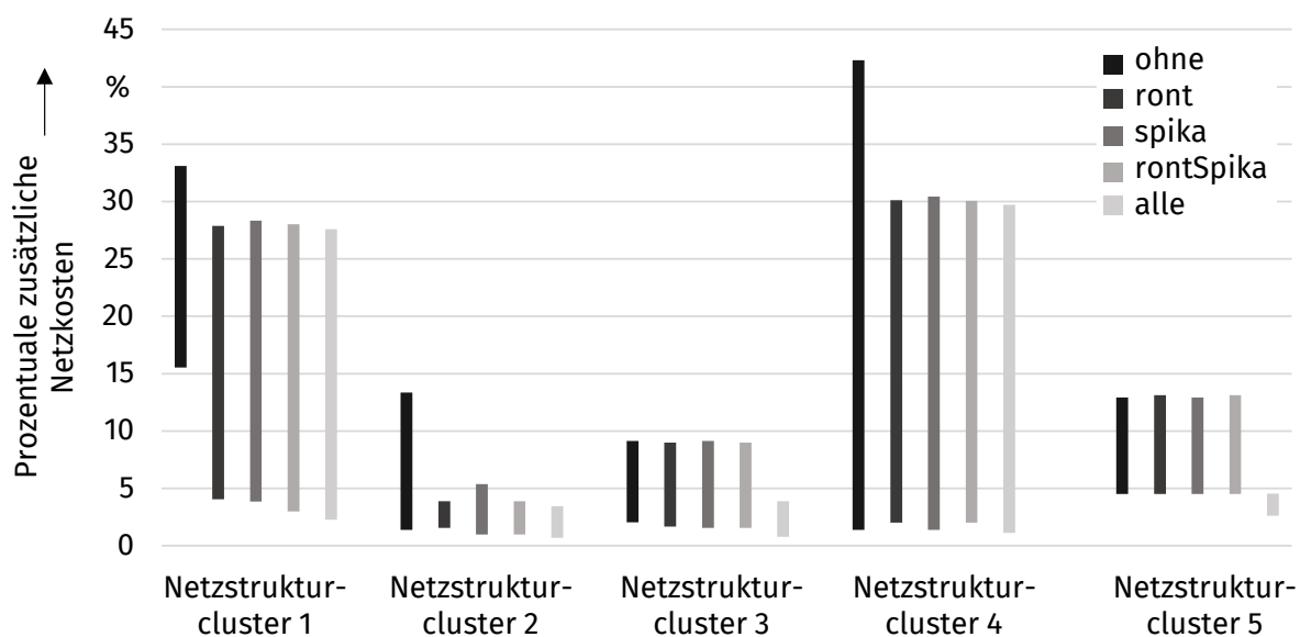
Abbildung 5.2-1: Bandbreite über die zusätzlichen Netzkosten im Verhältnis zur aktuellen Netzkosten aller Netzentwicklungscluster
