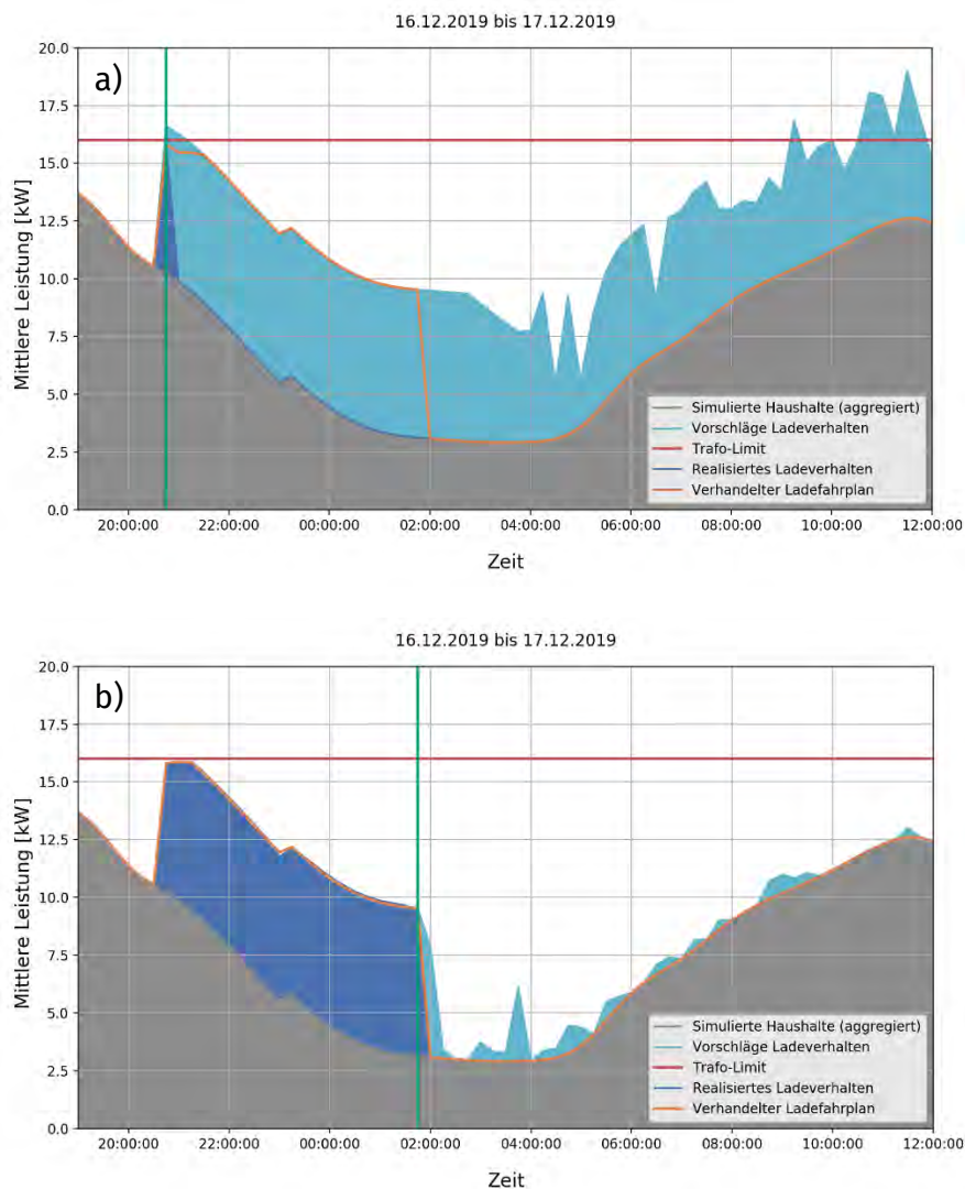
Abbildung 6.1-3: Vermeidung von simulierten Netzengpässen durch intelligentes G4M-Lademanagement
