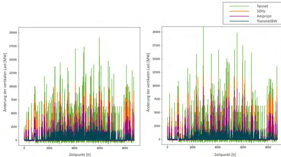
Abbildung 6.3-12: Jährlicher Verlauf der vertikalen Laständerung der vier deutschen Übertragungsnetzbetreiber für die Prognosehorizonte 1 Stunde (links) und 2 Stunden (rechts)
