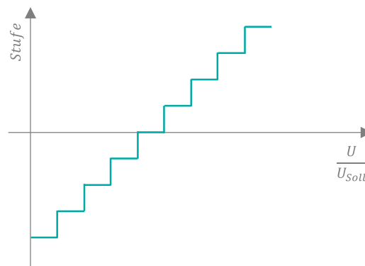
Abbildung 6.3-2: Regelungskennlinie eines automatisch stufbaren Transformators
