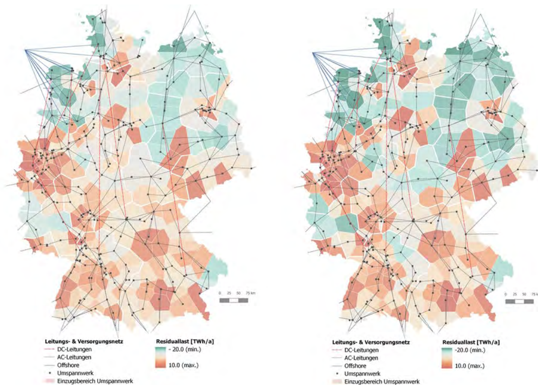
Abbildung 7.7-19: Verbleibende Residuallast je Übertragungsknoten in den Szenarien „Enera Worst Case 2030“ (links) und „Enera Best Case 2050“ (rechts)
