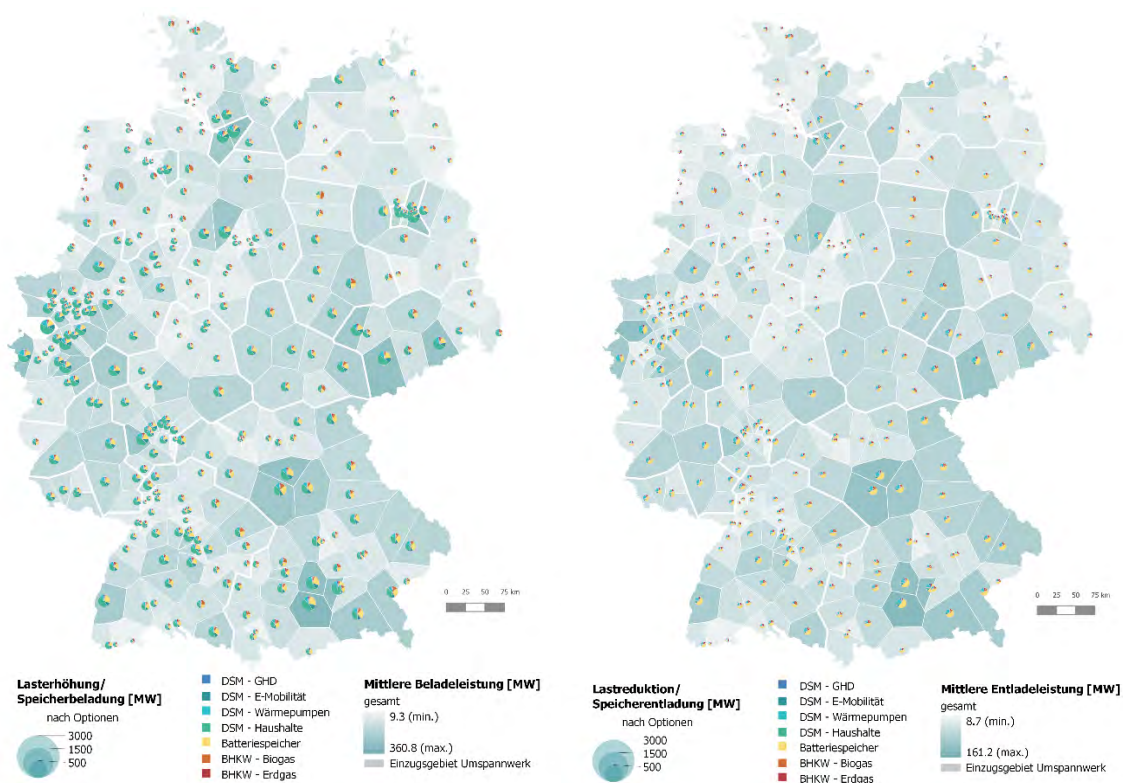
Abbildung 3.3-2: Verfügbares Potenzial dezentraler Flexibilitätsoptionen je Übertragungsnetz-knoten im Szenario „Enera Worst Case 2030“: mittlere Beladeleistung (links) und mittlere Entladeleistung (rechts)
