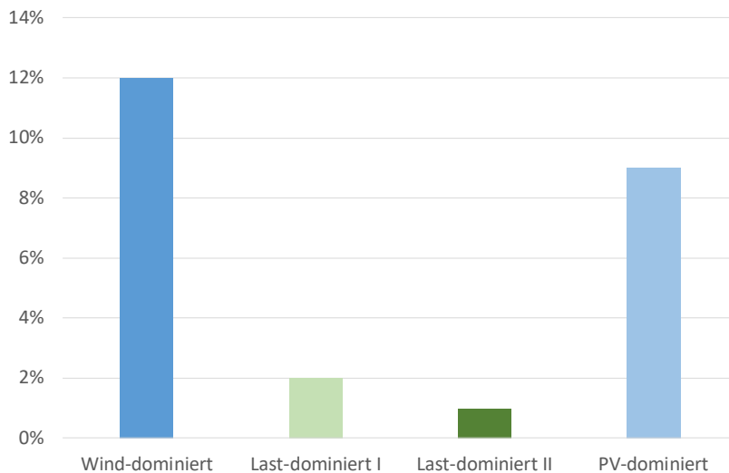
Abbildung 4.2-2: Mittlere Prognoseabweichung (normiert auf Transformator-Nennleistung MW/MWA)
