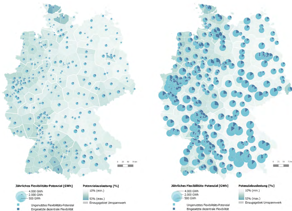
Abbildung 7.7-27: Nutzung des für den übertragungsnetzdienlichen Einsatz verfügbaren dezentralen Flexibilitätspotenzials in den Szenarien „Enera Worst Case 2030“ (links) und „Enera Best Case 2050“ (rechts)
