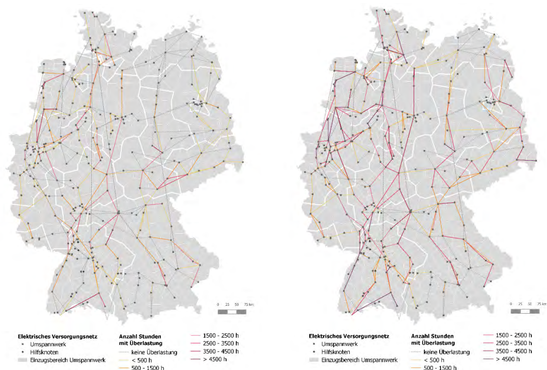
Abbildung 7.7-24: Anzahl der Stunden mit Netzüberlastung auf den einzelnen Leitungen in den Referenzszenarien „Enera Worst Case 2030“ (links) und „Enera Best Case 2050“ (rechts)
