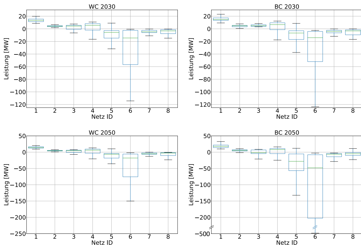
Abbildung 6.3-9: Leistungsflüsse über HS/MS-Umspannstation, Auswertung stündlicher Mittelwerte eines Jahres
