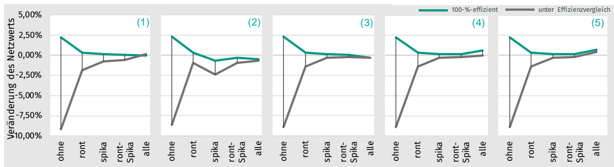
Abbildung 5.2-3: Ergebnis für die betriebswirtschaftlichen Bewertung des Netzentwicklungsclusters 1.4.
