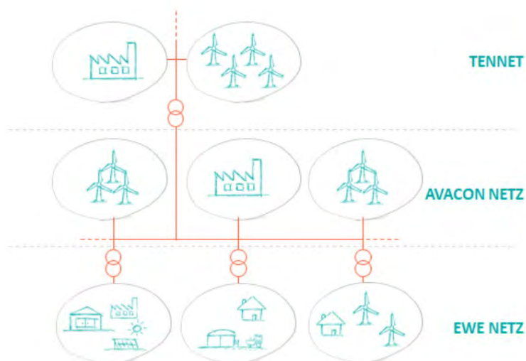
Abbildung 7.2-1: Marktgebiete über Spannungsebenen
