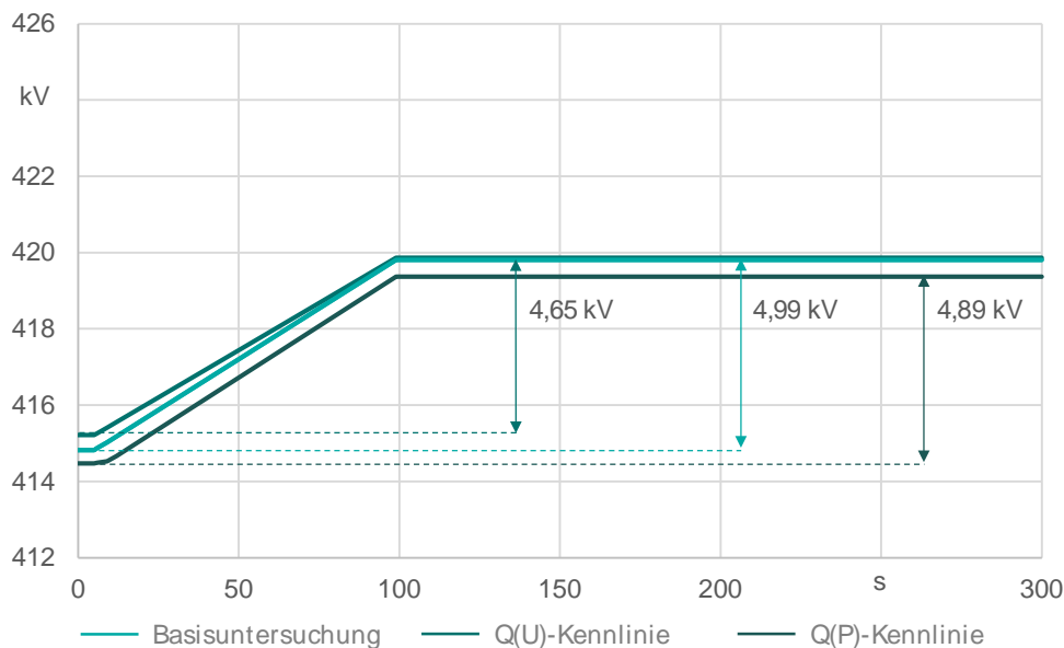
Abbildung 6.3-5: Spannungsverlauf am Fehlerort für Untersuchungsszenario 3
