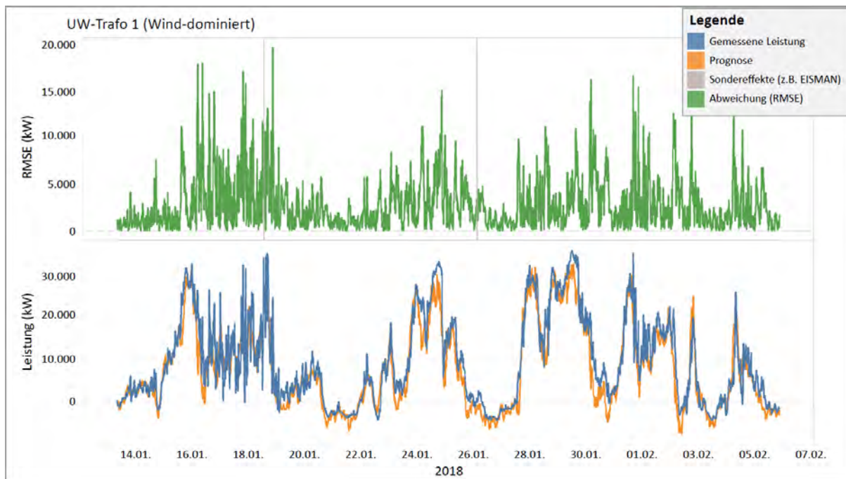
Abbildung 4.2-1: Beispielhafte Prognose für wind-dominierten UW-Transformator
