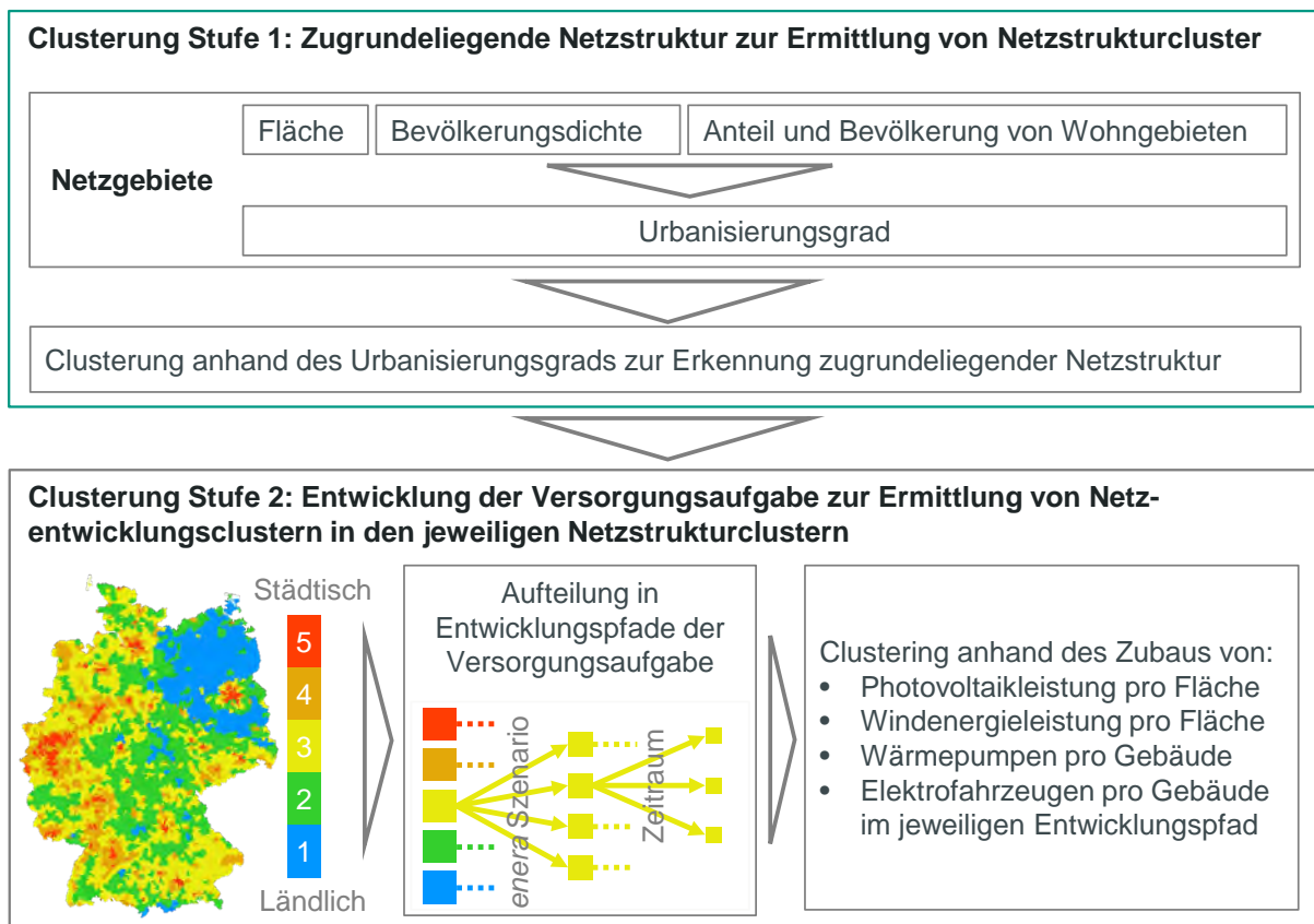
Abbildung 5.1-4: Verfahren der zweistufigen Clusteranalyse
