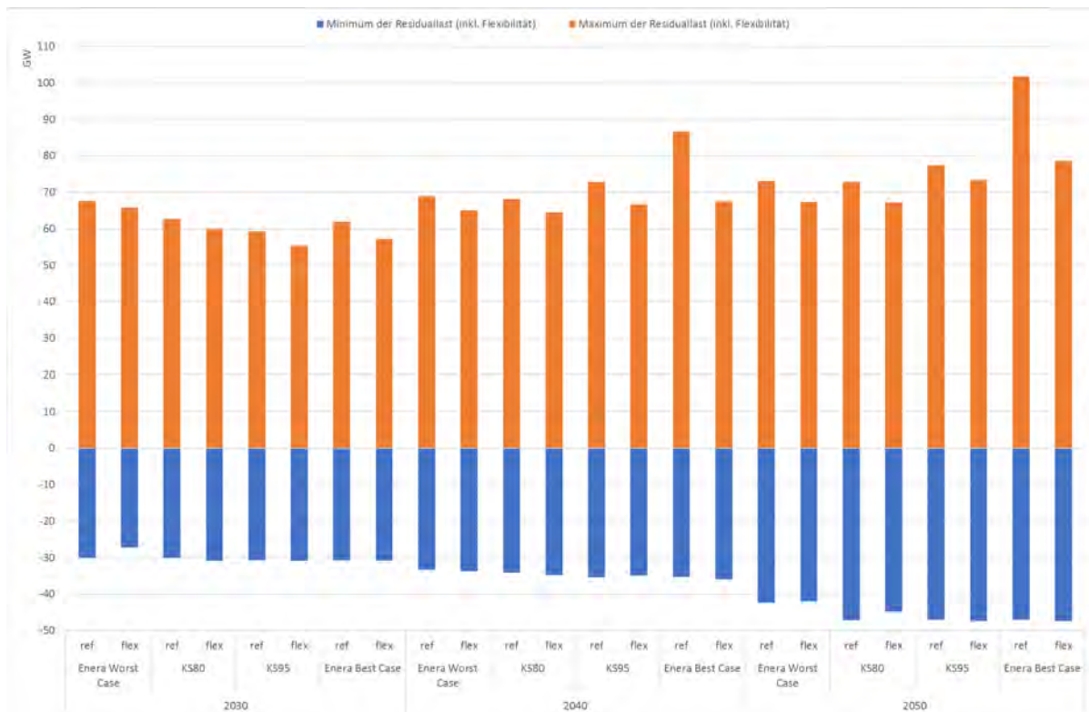
Abbildung 7.7-14: Maximum und Minimum der verbleibenden residualen Last in den enera Szenarien vor („ref“) und nach („flex“) dem strommarktdienlichen Einsatz der dezentralen Flexibilitätsoptionen
