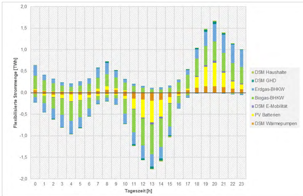
Abbildung 7.7-12: Einsatz der dezentralen Flexibilitätsoptionen im Tagesverlauf im „Enera Worst Case“ Szenario 2030
