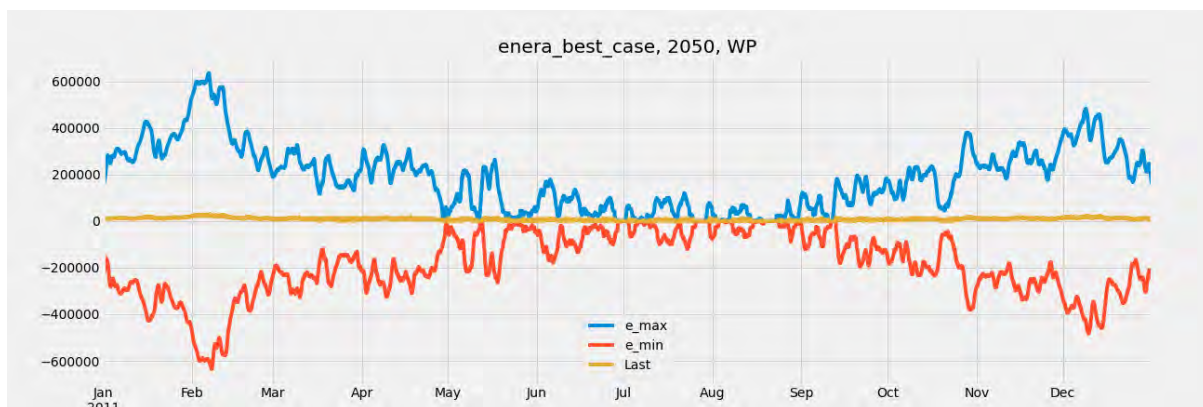
Abbildung 3.2-5: Die Füllstands-Grenzen eines fiktiven Speicher-Äquivalents für die gesamtdeutsche Nachfrage für Wärme aus Wärmepumpen im Jahresverlauf [MWh]
