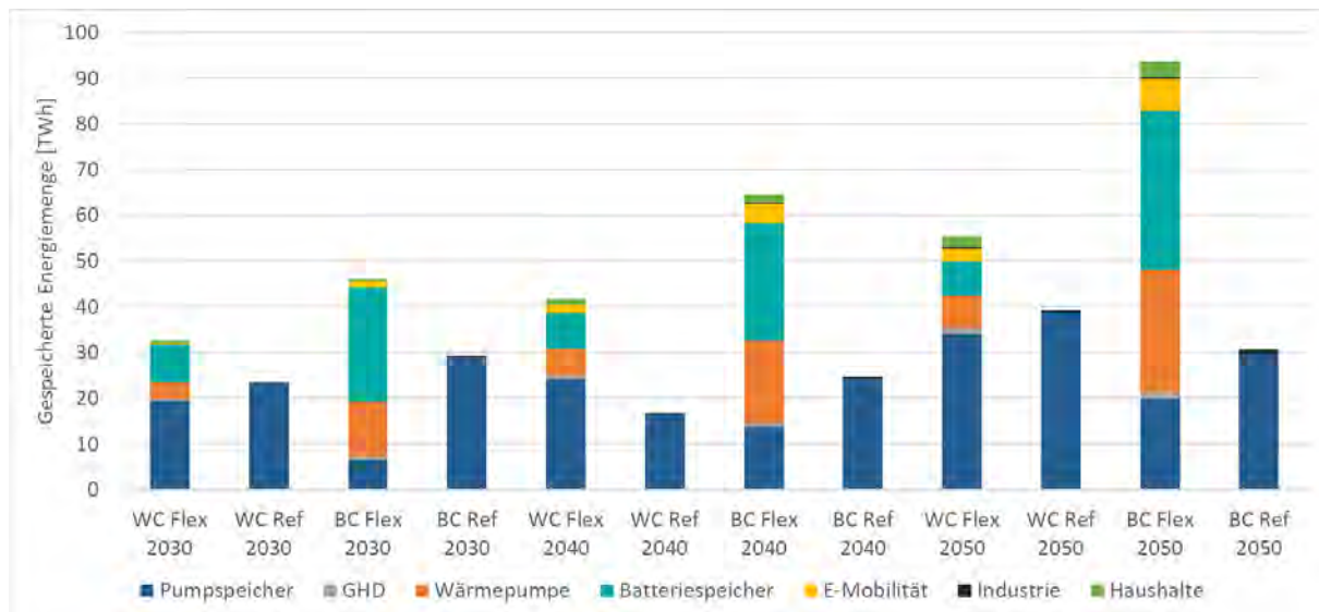
Abbildung 7.7-32: Gespeicherte Energiemenge der Flexibilitäten in TWh
