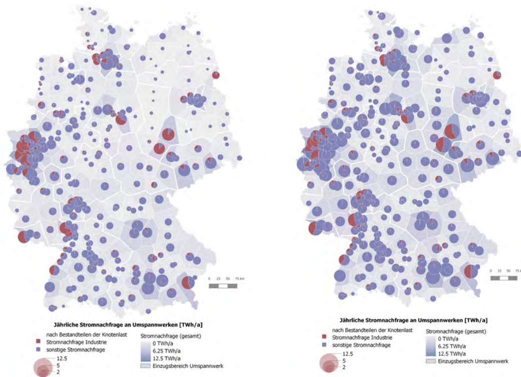
Abbildung 7.7-17: Regionalisierte Stromnachfrage je Übertragungsnetzknotten in den Szenarien „Enera Worst Case 2030“ (links) und „Enera Best Case 2050“ (rechts)
