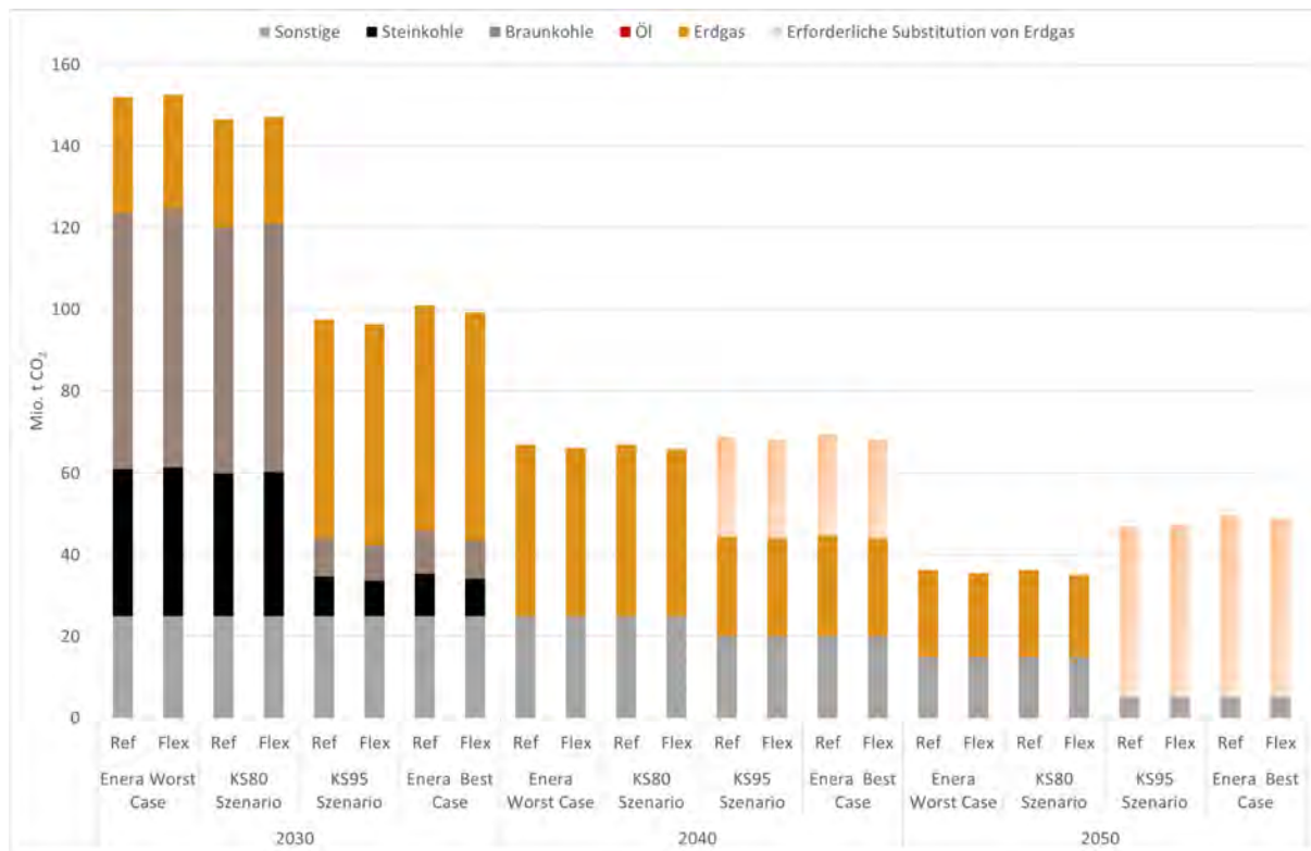
Abbildung 7.7-5: Brennstoffspezifische CO 2 -Emissionen der Stromerzeugung in Deutschland vor („ref“) und nach („flex“) dem strommarktdienlichen Einsatz der dezentralen Flexibilitätsoptionen
