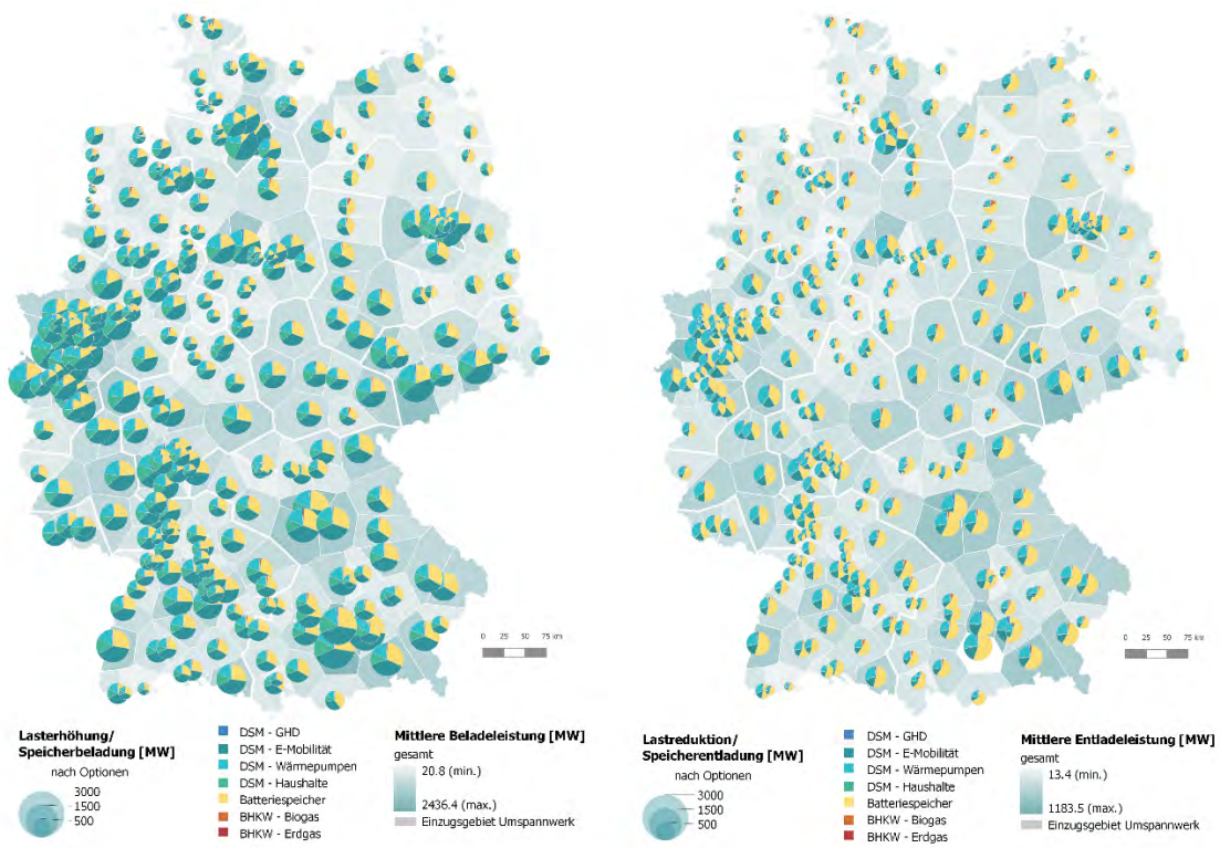
Abbildung 3.3-3: Verfügbares Potenzial dezentraler Flexibilitätsoptionen je Übertragungsnetz-knoten im Szenario „Enera Best Case 2050“: mittlere Beladeleistung (links) und mittlere Entladeleistung (rechts)
