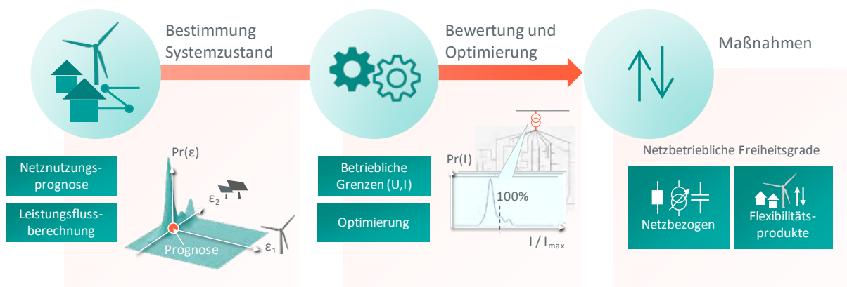
Abbildung 6.2-1: Übersicht des entwickelten Verfahrens zur Simulation des zukünftigen Netzbetriebs
