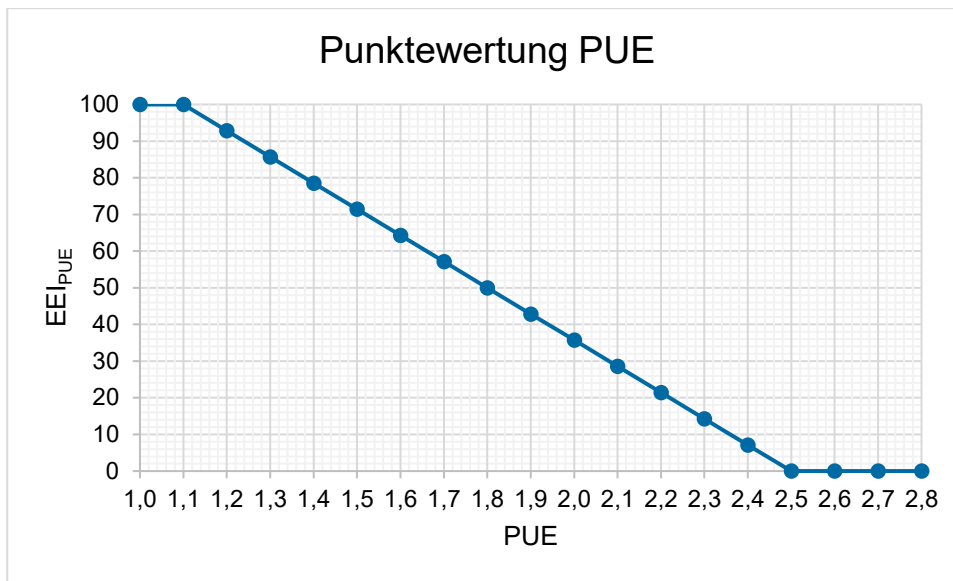
Abbildung 1: Energieeffizienzindex EEI_{PUE}
